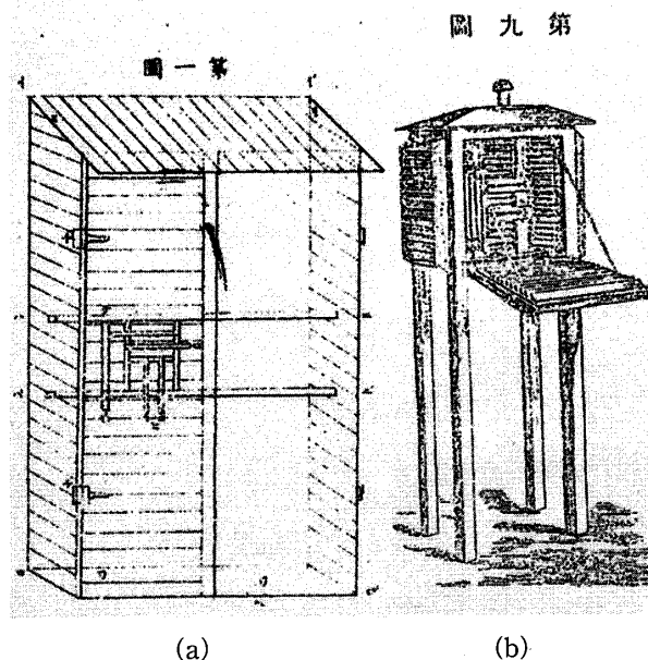
第1図 初期の百葉箱。(a) 1880年刊行「気象観測法」より。(b) 1886年制定公布「気象観測法」より。
