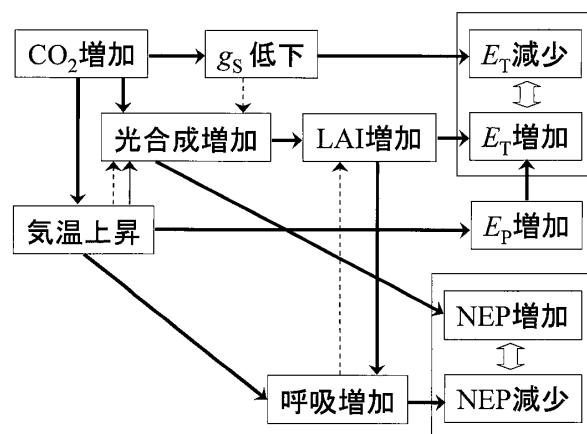
第2図 大気中CO 2 濃度の増加とそれにもなう気温の上昇が, 大気-陸域生態系の水・CO 2 交換におよぼす影響. ここでは主要な要因のみを, 矢印で示した (実線: プラスの効果, 破線: マイナスの効果). 気温上昇が光合成に及ぼす効果は, 条件によりプラスまたはマイナスとなる. g_s : 気孔コンダクタンス, E_T : 蒸散量, E_p : ポテンシャル蒸発量, LAI: 葉面積指数.
