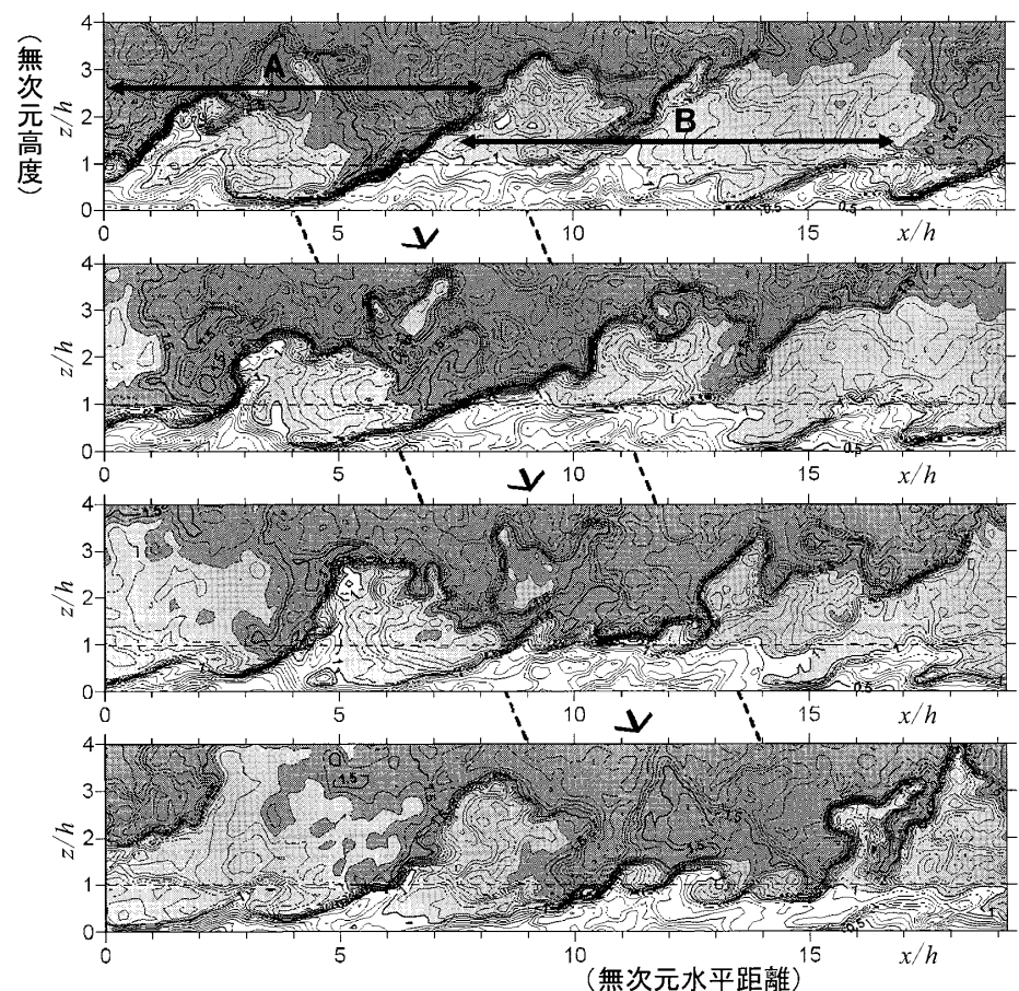
第 3 図 LES (Large Eddy Simulation) によって計算された中立条件における群落内外のスカラー量 (\chi - \chi_c) / (\chi_h - \chi_c) の鉛直断面の時間変化 18) 。 \chi はスカラー量を表し、添字 c と h で地表面ならび群落上端における平均値を示している。各コマの時間間隔は 0.8 h / U_h ( h : 群落上端高度, U_h : 群落上端の平均風速)。最上図において、高速ストリーク (A) と低速ストリーク (B) の間にスカラー量の不連続 (微細前線) が確認できる (矢印は微細前線の動き)。
