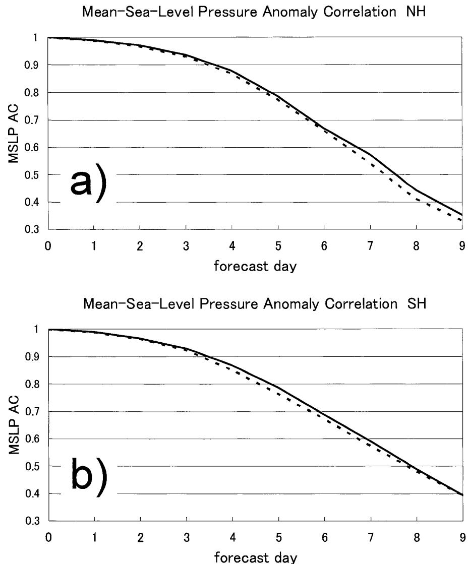
第6図 海面気圧のアノマリー相関（2007年10月の月平均）。a) 北半球とb) 南半球。実線は新全球モデル，点線は旧全球モデルの成績。値が大きいほど解析場と予報場のパターンが類似している（予報が正しい）ことを意味する。
