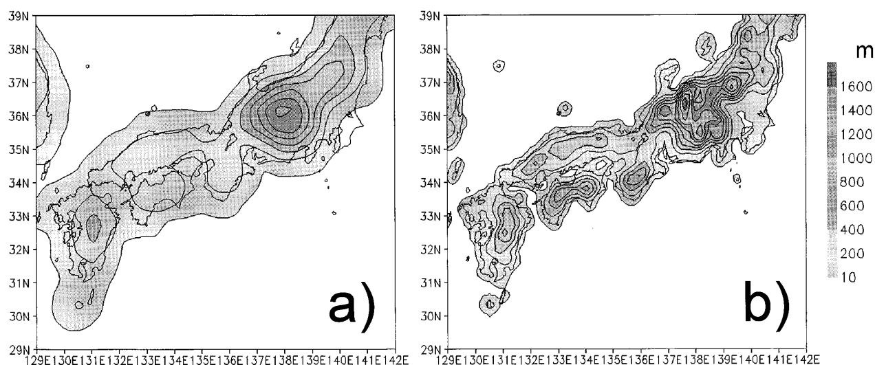
第2図 全球モデルの地形標高分布. a) 旧モデル, b) 新モデル.
