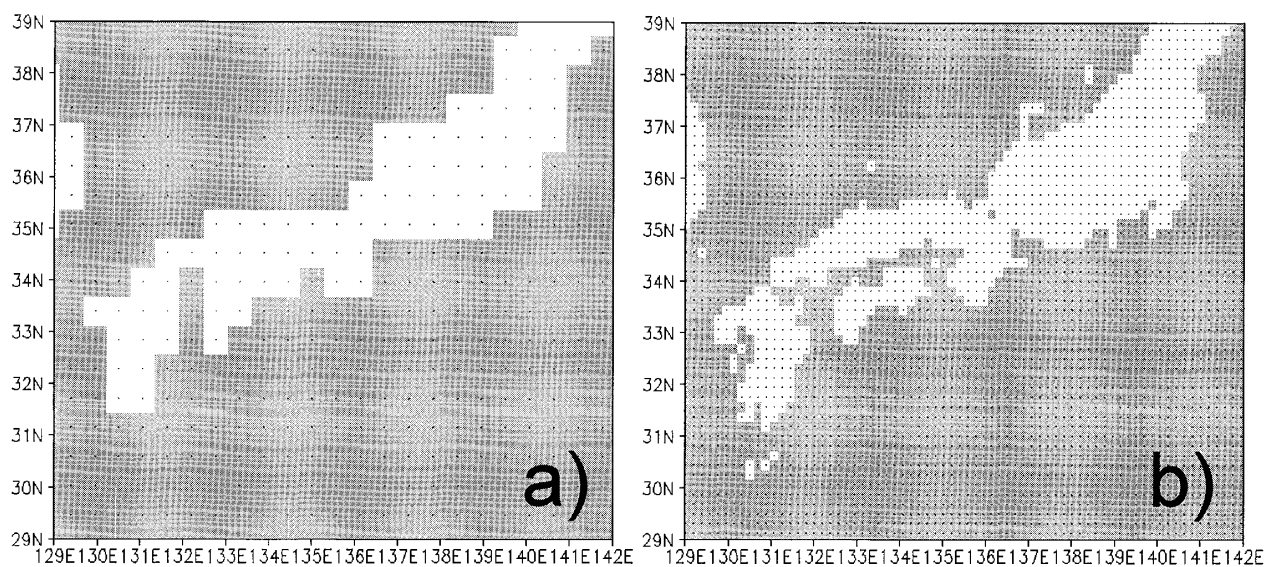
第1図 全球モデルの海陸分布. a) 旧モデル, b) 新モデル.
