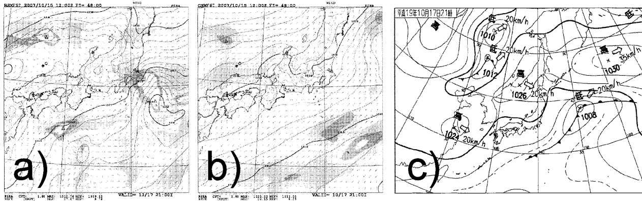
第5図 領域モデルによる“にせ”の低気圧の予報例。a) 領域モデル予報，b) 新全球モデル予報，c) 実況天気図。ハッチは6時間降水量 (mm)，等値線は海面気圧 (hPa)。実際には，関東地方の南東海上に低気圧は発生しなかった。(aとbは関東付近を拡大して見やすくしてあり，cとは描画領域が異なっていることに注意。)
