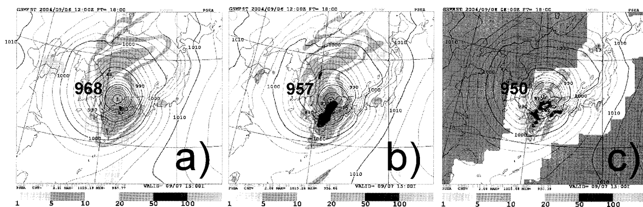
第4図 全球モデルによる2004年台風第18号の予報。a) 旧モデル予報、b) 新モデル予報、およびc) 実況。ハッチは6時間降水量 (mm)、等値線は海面気圧 (hPa)、図中の数値は台風中心の気圧値 (hPa)。
