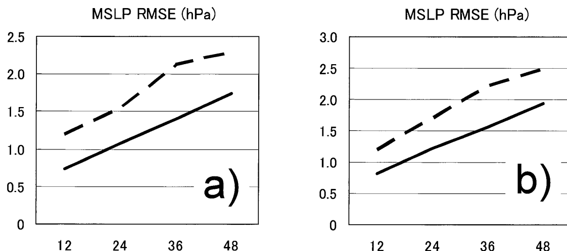
第7図 日本付近における海面気圧の平均二乗誤差の平方根 (Root-Mean-Square Error). a) 2004年8～9月, およびb) 2005年12月～2006年1月の平均. 実線は新全球モデル, 破線は領域モデルの成績. 横軸は予報時間.
