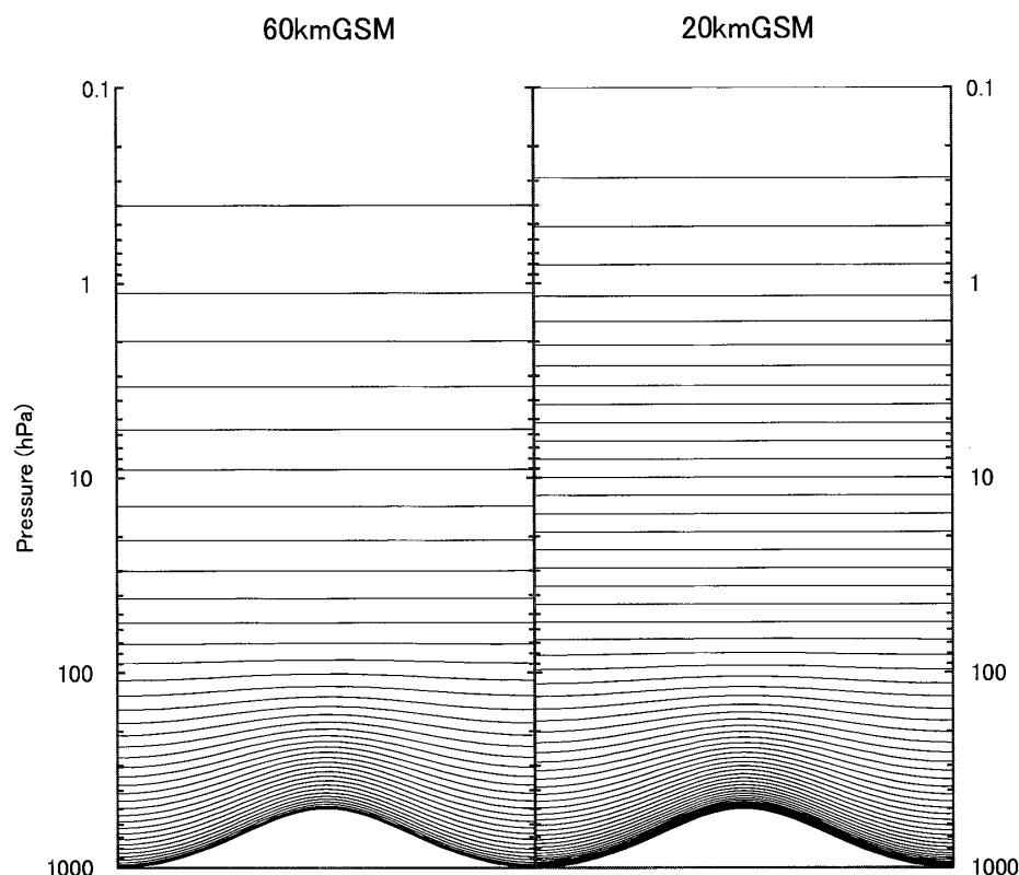
第3図 全球モデルの鉛直気圧層配置の比較.
