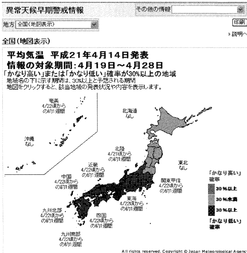
第3図 気象庁HP「異常天候早期警戒情報」の全国地図表示の例（気象庁HPより転載）。平成21年4月17日に発表した情報文の地図表示結果。関東甲信、北陸地方から奄美地方までの広い範囲を、凡例にある「かなり低い」確率30%以上のパターンで塗りつぶし、これら地方で「かなりの低温」となる可能性が高いことを示す。また、その警戒期間も各地域名そばに添えている。
