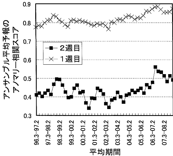
第5図 アンサンブル数値予報の成績の経年変化。予測対象は1か月EPSによる日本周辺領域（北緯20～60度，東経100～170度）500 hPa 面高度。横軸は，予報毎に算出した検証スコアの平均期間（1年間）を表し，左端が1996年3月からの1年間，右端が2007年12月からの1年間と3か月刻み。縦軸はアノマリー相関スコアを表す。アノマリー相関スコアとは，予測と実況の偏差パターンが完全に一致（反転）すると最大値の1（最小値の-1）となる量で，0は無相関を意味する。■印と×印の折線はそれぞれ2週目と1週目のスコア。
