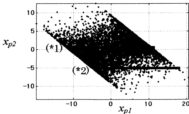
第 3 図 PCA によって得られた主成分 x_{p1}(t) , x_{p2}(t) の散布図.
