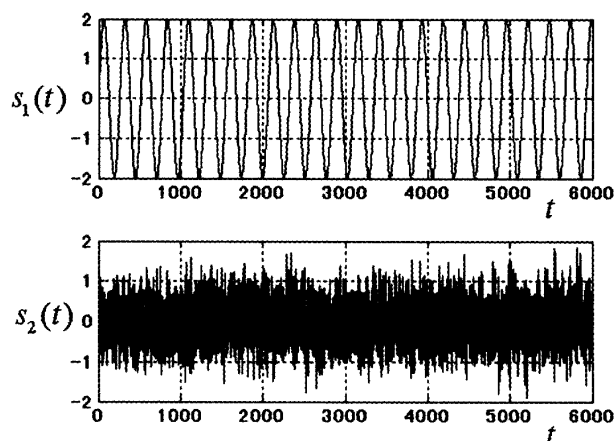
第1図 人工的な源信号 ( s_1(t) : 正弦波, s_2(t) : 正規乱数)。
