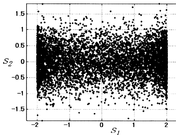
第2図 源信号 s_1(t) , s_2(t) の散布図 (同時確率密度分布)。
