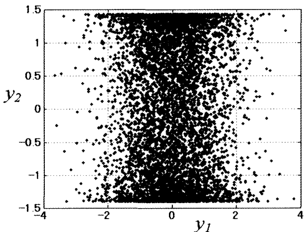
第 4 図 ICA によって推定された源信号 (独立成分) の散布図.
