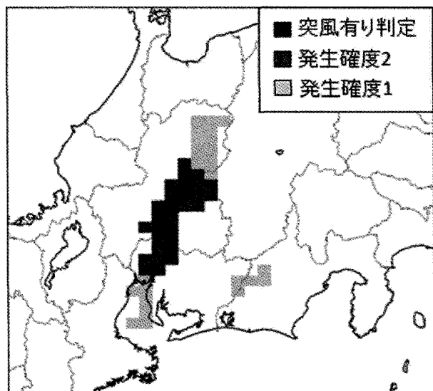
第7図 発生確度2と竜巻注意情報の関係。
