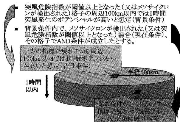
第3図 突風の総合判定の概要。
