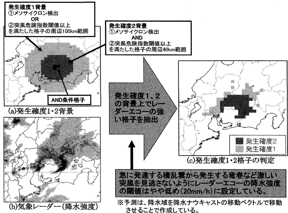
第 4 図 発生確度 1・2 の作成方法.
