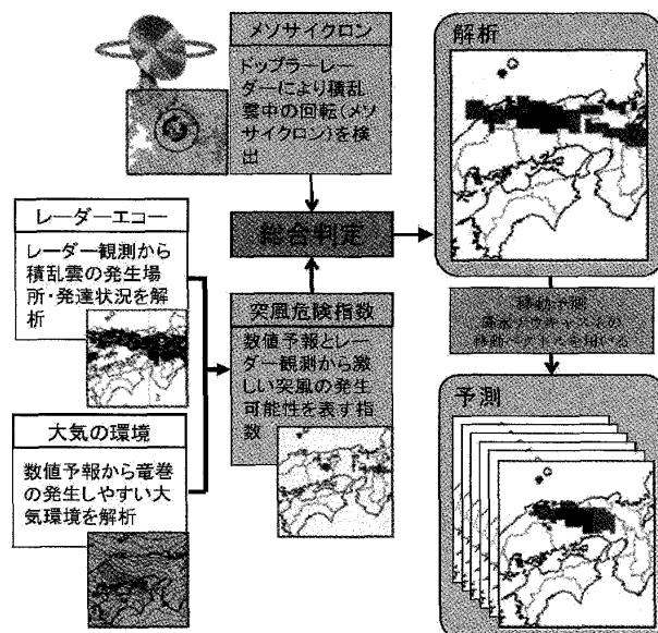
第2図 竜巻発生確度ナウキャストの解析・予測技術。
