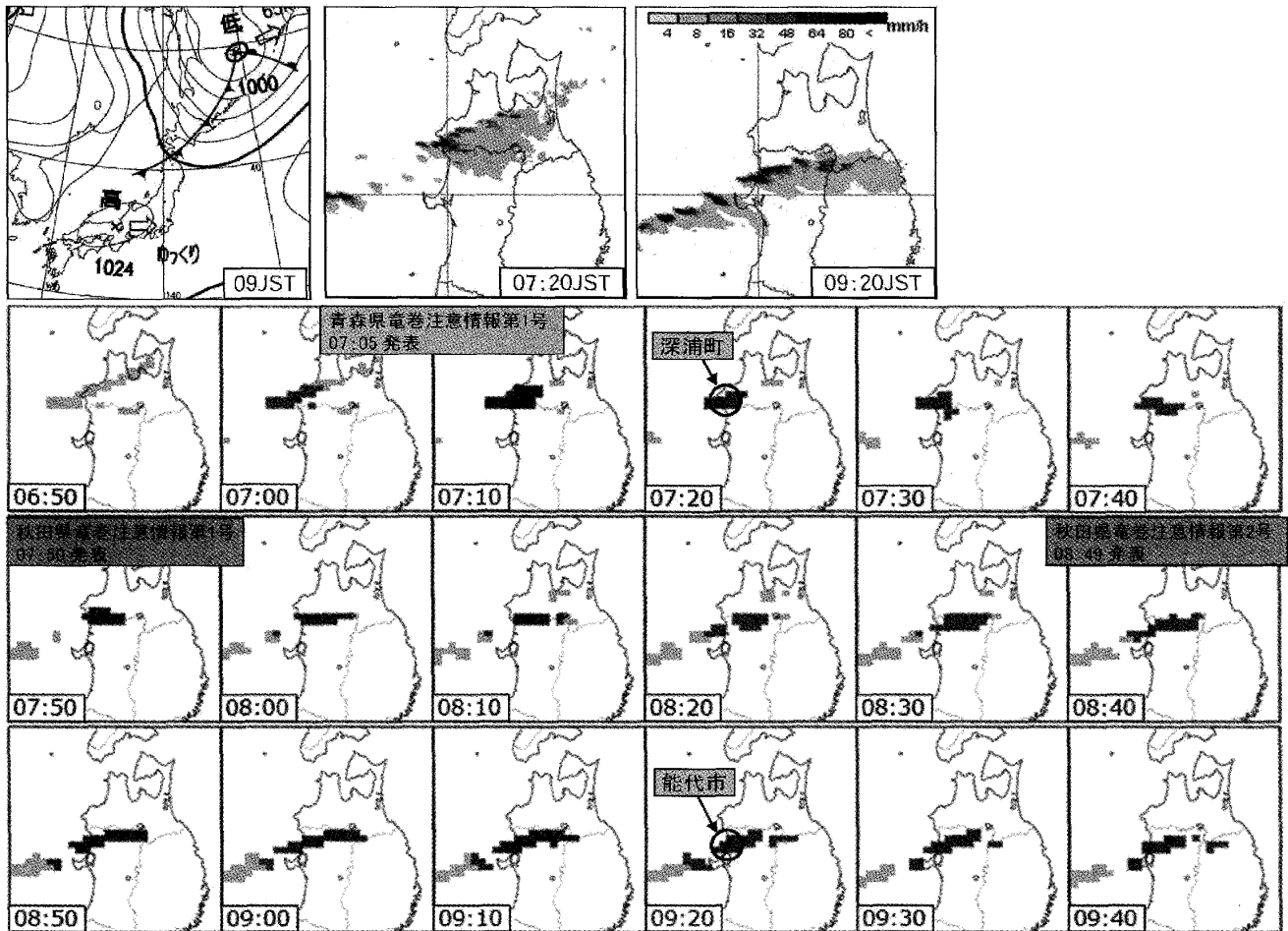
第6図 竜巻発生確度ナウキャストの解析事例。2009年10月30日に青森県深浦町で発生した竜巻（07:20頃，F0），秋田県能代市で発生した竜巻（09:20頃，F1）の解析。上段左：地上天気図，上段中・右：全国合成レーダー画像（降水強度），下段：竜巻発生確度ナウキャスト解析（濃い灰色は発生確度2，薄い灰色は発生確度1を表す）。
