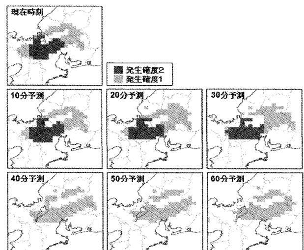
第 5 図 竜巻発生確度ナウキャストの予測事例 (2007年 7 月12日10時20分初期時刻). 40 分予測で発生確度 2 が消滅しているのは, 発生確度 2 背景の判定がでてから 1 時間が経過したため.
