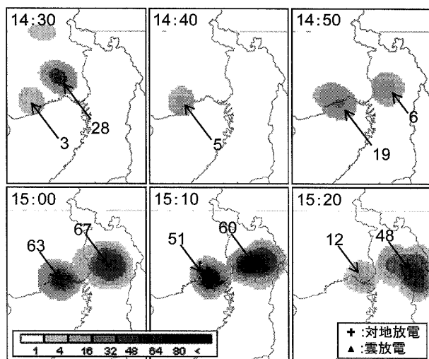
第6図 レーダー雷解析の事例 (2009年5月24日 兵庫県・大阪府). 14時30分から15時20分のレーダー雷解析の指数(0~100)の値と, LIDEN で検出した対地放電・雲放電.
