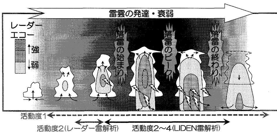
第2図 雷雲の発達過程と活動度の対応。
