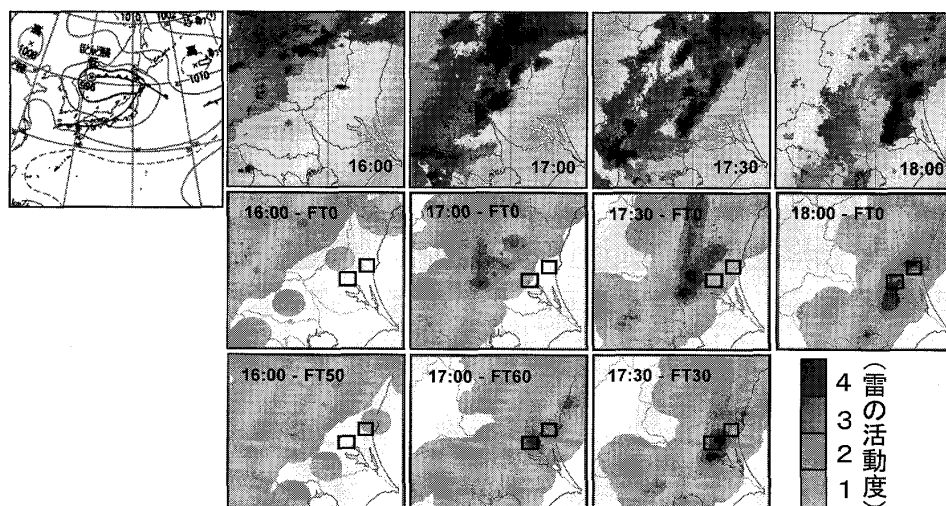
第10図 雷ナウキャストの予測事例。2008年8月19日茨城県の雷ナウキャストの解析・予測事例。左上は15時地上天気図。上段はエコー強度、中段は雷ナウキャストの解析、下段は雷ナウキャストの予測。時刻は初期値、FTの右の数字は予測時間（分）を表す。黒枠は、雷災害の発生した水戸市と石岡市。
