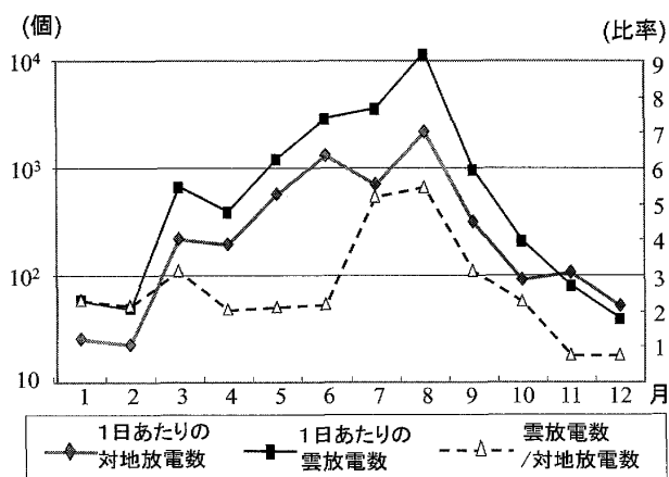
第3図 月別の放電数と放電種別の比率。2007年の放電数を月別に集計し、月の日数で割って1日あたりの放電数とした値（左軸、ログスケール）。また、破線は対地放電に対する雲放電の比率を示したもの（右軸）。
