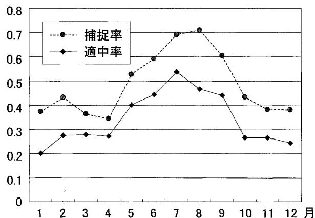
第9図 適中率・捕捉率。雷ナウキャストの30分予測の活動度2以上の月毎の適中率・捕捉率。雷ナウキャストの解析値（活動度2以上）を検証の真値とした。適中率は、30分予測で活動度2以上となる格子に対して、その格子から半径5 km以内に真値の格子がある割合。捕捉率は、活動度2以上を解析した格子に対して、その格子から半径5 km以内に、30分過去の時刻を初期値とした予測で活動度2以上を予測した格子の存在する割合。
