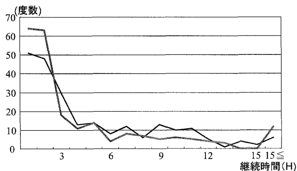
第4図 関東地方夏季雷（7・8月）と北陸地方冬季雷（11・12月）の継続時間ごとの事例数の度数分布。1時間区切りで集計。黒線は関東夏季、灰色線は北陸冬季。2005～2008年の集計で、対象とする関東夏季・北陸冬季の面積及び集計日数はほぼ等しい。対象地域において10分単位で30分連続で放電を検知した時刻から、30分連続で放電を検知しなくなった時刻までを一つの事例として扱った。
