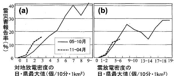
第5図 放電密度と雷災害報告率の対応。日・県単位の対地放電(a)、雲放電(b)の放電密度最大値と雷災害報告率（雷災害報告のあった日数の割合）の関係。(a)と(b)の縦軸のスケールは同一。横軸のスケールは、日最大放電密度の出現する頻度が同程度になるよう調整した。つまり、対地放電の日最大放電密度9以上の発現する頻度と、雲放電の日最大放電密度19以上の発現する頻度は同程度である。統計期間は2005～2007年。ここで「雷災害報告」とは、気象官署が県単位で一連の擾乱ごとに取りまとめる気象災害報告のうち、落雷によるものである。
