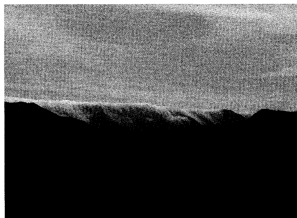
第1図 上越国境に発生した滝雲 (1). 2007年9月2日09時34分に撮影。撮影方向は第3図の地点Aから東方向。
