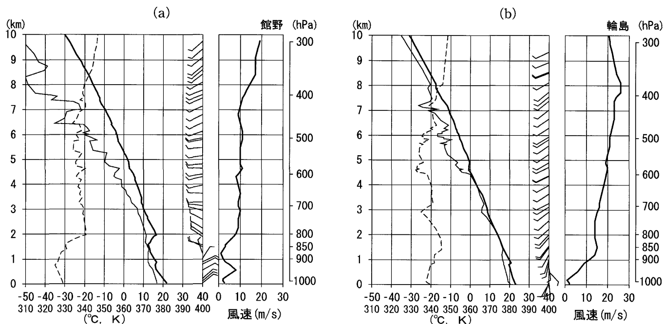
第7図 2007年9月2日09時(日本時間)の館野(a)と輪島(b)のエマグラム. 矢羽根は上を北とした風向. 各図の右側の実線は風速, 左側の太実線は気温, 細実線は露点温度, 破線は相当温位.
