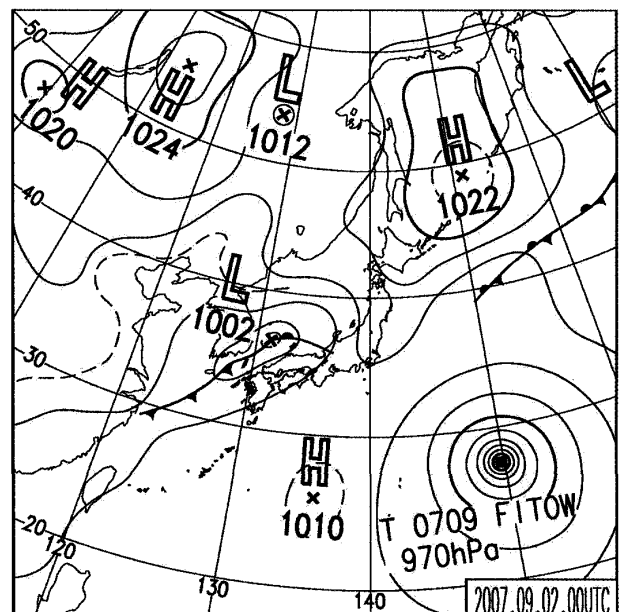
第4図 2007年9月2日09時（日本時間）の地上天気図。
