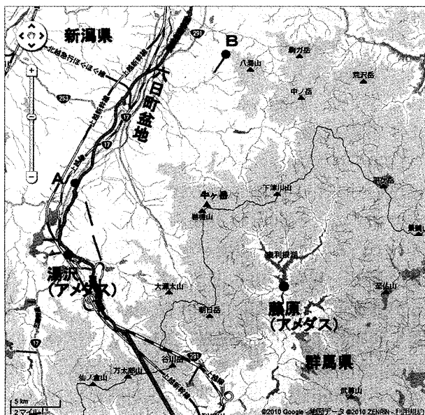
第3図 滝雲の撮影地点と新潟県南魚沼市周辺図。Google 地図より。A, B はそれぞれ第1図、第2図の撮影地点。
