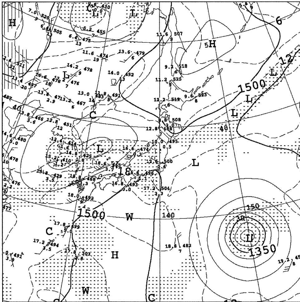
第5図 2007年9月2日09時（日本時間）の850hPa天気図。
