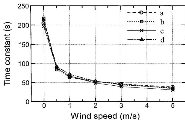
第4図 温度計の時定数と通風速度との関係。
