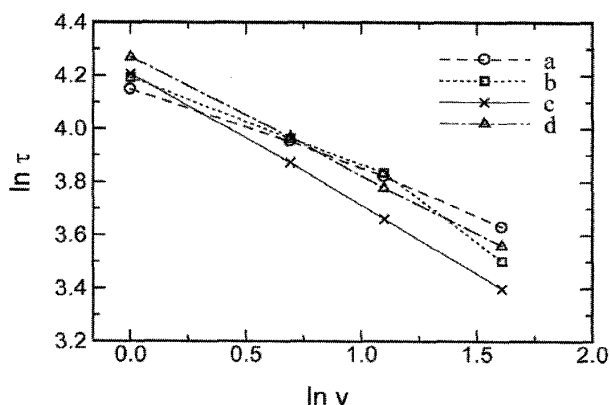
第6図 温度計の時定数と通風速度との関係(式(6)).
