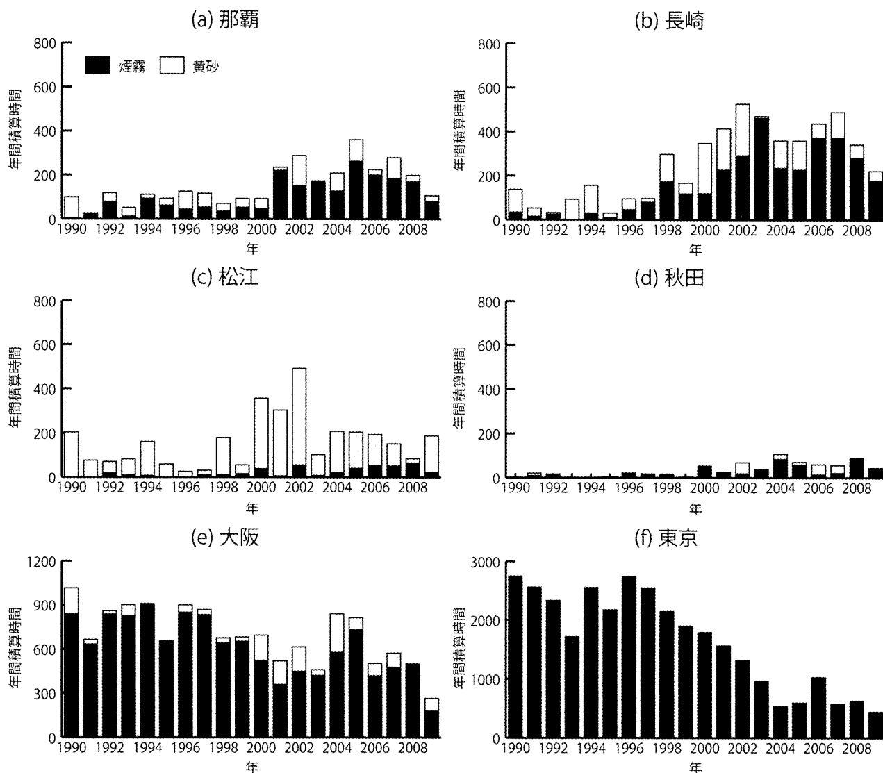
第1図 気象庁による1990～2009年の年別の煙霧（黒）と黄砂（灰色）の積算観測時間。
