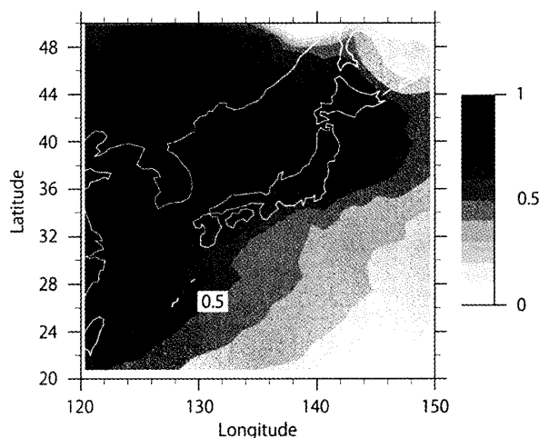
第2図 SPRINTARSによるモデル最下層の消散係数の合計に対する人為起源エアロゾルの消散係数の比率（2006年平均）。
