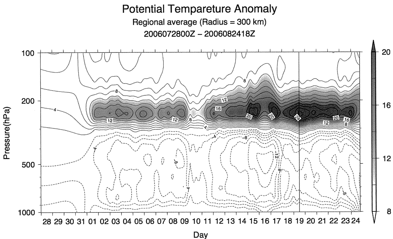
第3図 2006年7月末から8月にかけての北極低気圧中心から半径300 km 平均した温位のアノマリの鉛直時間断面（2 K ごと、点線は負値）。対流圏は寒気核、下部成層圏は暖気核になっている。
