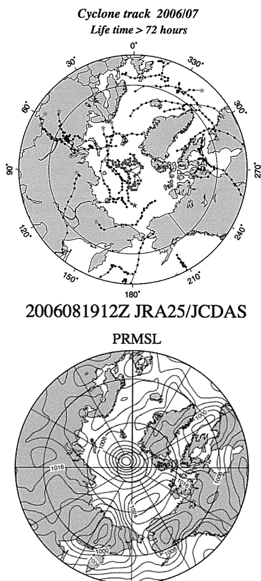
第1図 (上) 2006年7月に北極圏で出現した低気圧の経路。起点の星印が発生位置を示す。中央の星印からの経路 (灰色) が北極低気圧の例で、7月28日に発生しひと月間迷走したもの。(下) 8月19日の海面気圧の分布 (4 hPa ごと)。北極点付近の低気圧が北極低気圧。
