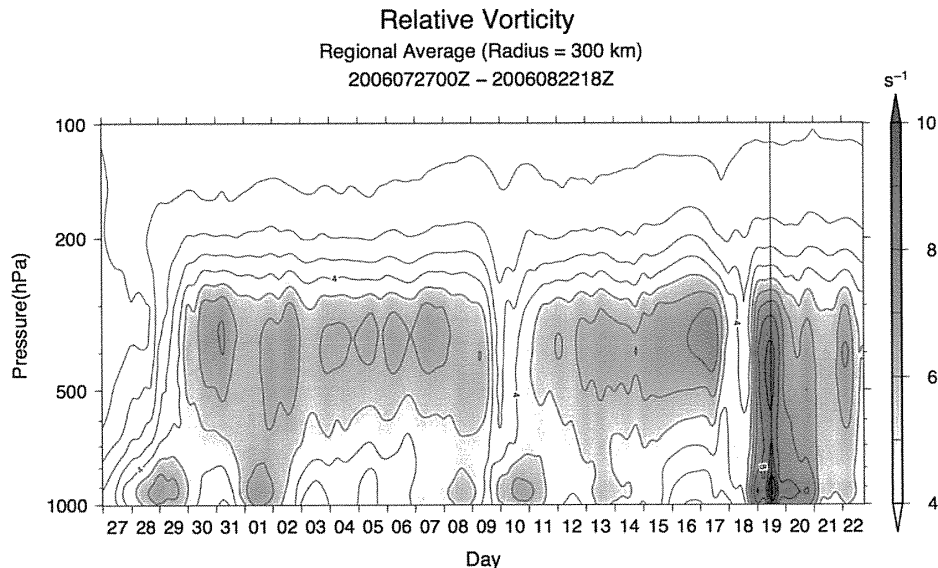
第2図 2006年7月末から8月にかけての北極低気圧中心から半径300 km 平均した相対渦度の鉛直時間断面。相対渦度は気圧 (p/p_s)^{1/2} \times 10^5 で正規化してある。最盛期は8月19日。
