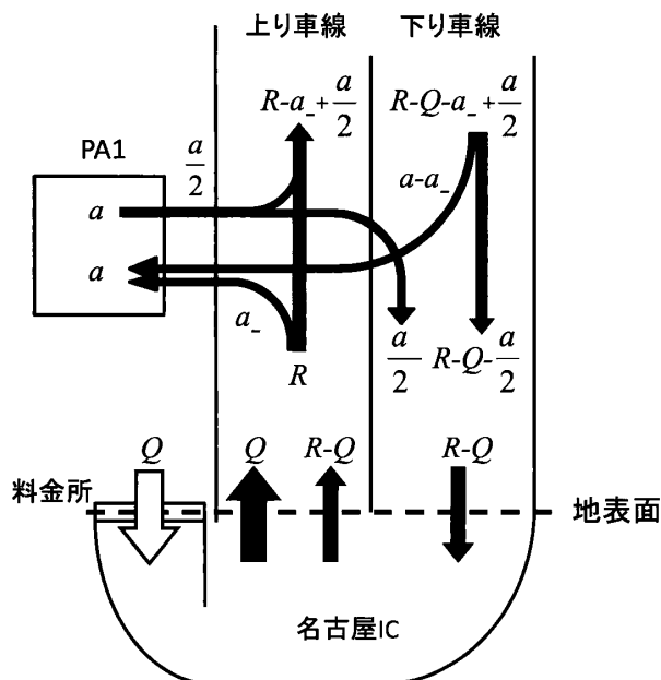
第1図 地表面（名古屋IC）と名古屋ICの次のPA（以下「PA1」という）での放射フラックス（車の流れ）。白抜き矢印は太陽放射、黒矢印は赤外線に対応する。 R は名古屋ICから上り車線に入る車のフラックス、 a は上り車線および下り車線からPA1に入る（吸収される）車のフラックスの合計であり、入ったのと同数 a の車がPA1を出て、その半分（ a/2 ）が上り車線に、残り半分が下り車線に入る。名古屋・東京間で、PAが1か所しかない（下り車線でPAに到達する車はない）とした木村(2012)の第2図と異なり、PAが無限に密にある状態を表現しており、上り車線からは a_+ 、下り車線から a-a_+ の車がPA1に入る。 a および a_+ はPAの位置 \tau(=\tau_0'-\tau') の関数であり、PA1の位置を \tau_1 として、 a(\tau_1) などと表記するべきであるが、簡単のためここでは単に a などと表記した。
