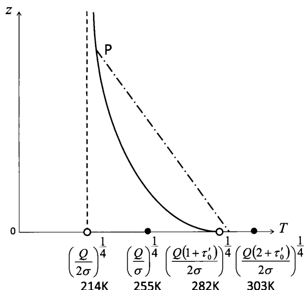
第4図 放射平衡で得られる気温 T の高度分布 (概念図). 温室効果気体が存在する大気 (実線) と温室効果気体が存在しない (無限少) 大気 (破線) について示す. あわせて地表面温度を黒丸で示す. 第3図bと同様, 温室効果気体の密度は地表面から高度ともに指数関数的に減少することを考慮している. 横軸下の数値は温室効果気体の光学的厚さ \tau_0' を2とした場合の温度であり, ほぼ現実大気 の値を説明する. 一点鎖線は対流が生じた場合の気温分布を概念的に示したものである. 実線の曲線と斜めの一点鎖線の交点 P より下層が対流圏, 上層が成層圏になぞえられる.
