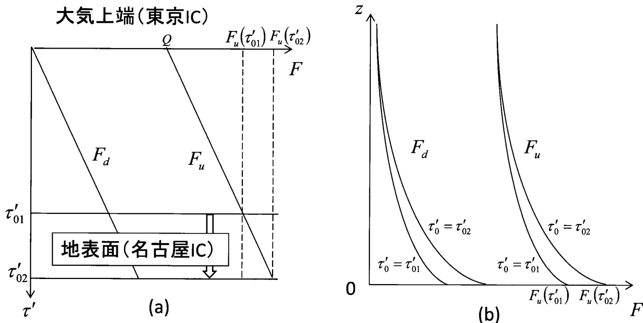
第3図 温室効果気体の光学的厚さが \tau'_{01} から \tau'_{02} に増加した場合の長波放射フラックス F の変化の概念図。(a) 東京 IC から名古屋 IC までの光学的厚さの増加に伴い地表面 (名古屋 IC) はグラフ上で \tau'_{01} から \tau'_{02} に移動する。光学的厚さの増加に比例して、地表面上向き放射フラックス F_u(\tau'_0) は増大する。(b) 高度分布で示したもの。温室効果気体の密度が地表面から高度とともに指数関数的に減少することを考慮している。
