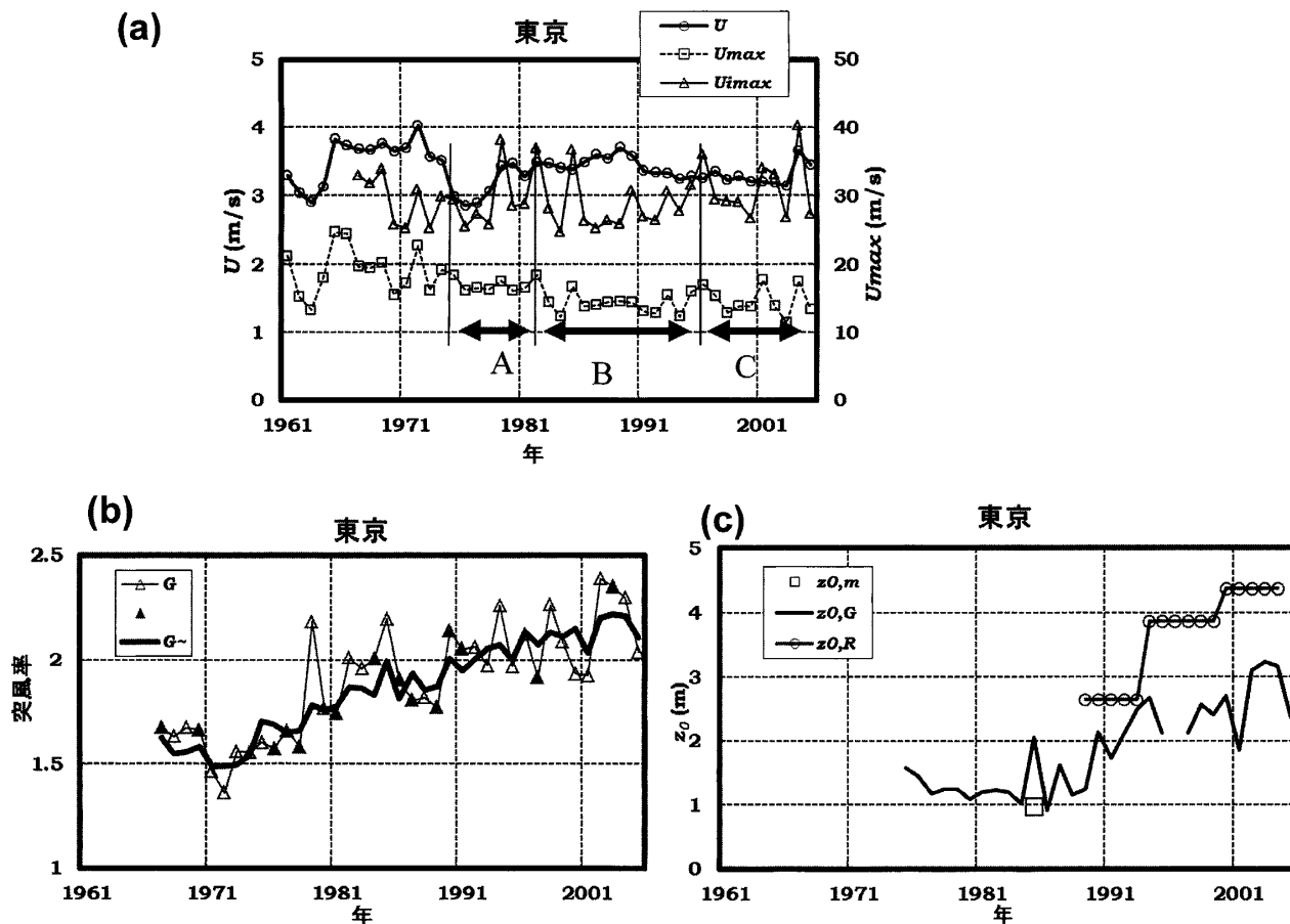
第1図 東京（気象庁大手町観測露場）における長期変化。(a) 平均風速，年最大風速および年最大瞬間風速，A，B および C はそれぞれ旧型，80型および95型の観測期間に対応，(b) 年突風率と平滑化年突風率， \triangle は年最大風速と年最大瞬間風速が同一日に発生， \blacktriangle 印は異なる日に発生，(c) 幾何学的粗度，突風率粗度およびロスビー数粗度。
