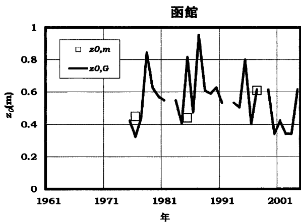
第2図 函館における突風率粗度 z_{0,G} の年々変化と1976年，1985年および1997年各年の幾何学的粗度 z_{0,m} 。
