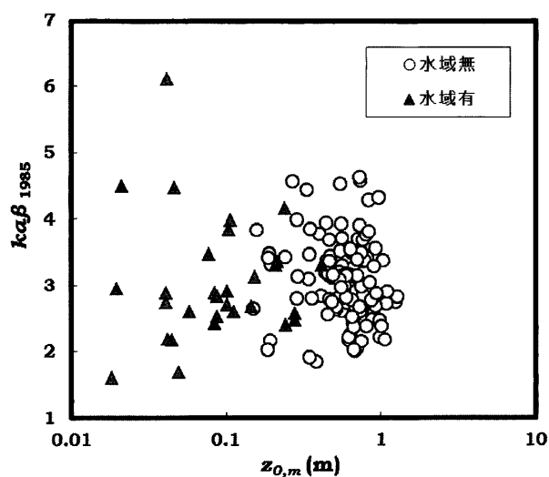
第3図 日本の気象官署153箇所の ka\beta_{1985} の粗度依存性。 z_{0,m} は1985年段階の幾何学的粗度から求めた風向別粗度の相乗平均値。 \blacktriangle 印は，湖沼，河川敷および海水域が90%以上占める方角がある地点である。
