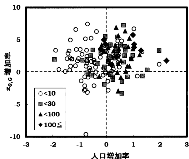
第5図 日本の気象官署151箇所における1975年から2004年の間の突風率粗度 z_{0,G} の増加率と1980年から2000年の間の人口増加率の関係。単位は%/年、マークは人口（万人単位）で分類。
