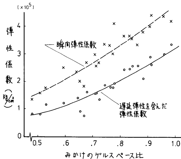
図12 みかけのゲルスペース比と弾性係数の関係
