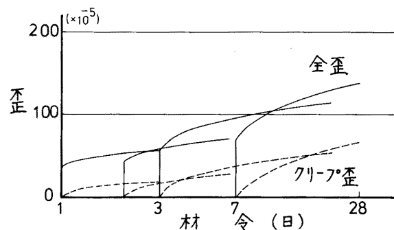
図4 荷重変化がない場合の歪量
