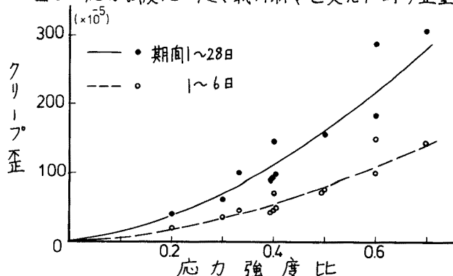
図7 応力強度比とクリープ歪との関係
