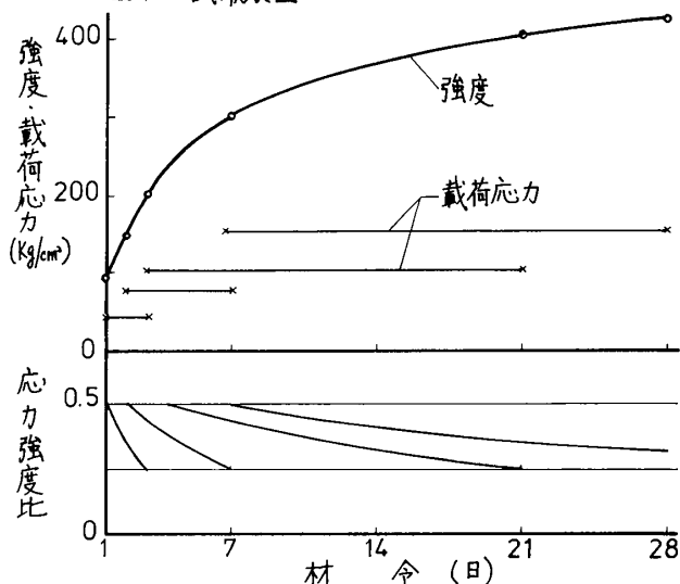
図2. 強度・載荷応力 応力強度比の変化
