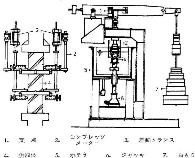
図1 試験装置
