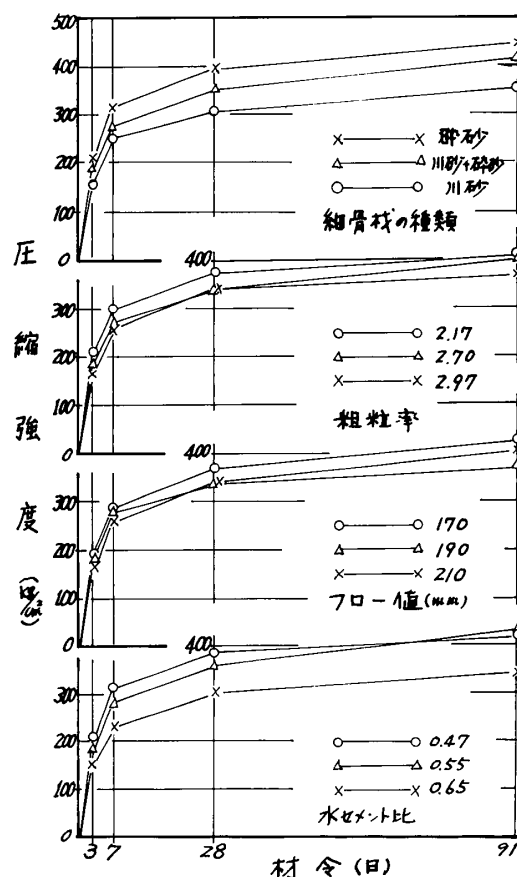
図4 要因別 材令と圧縮強度の関係
