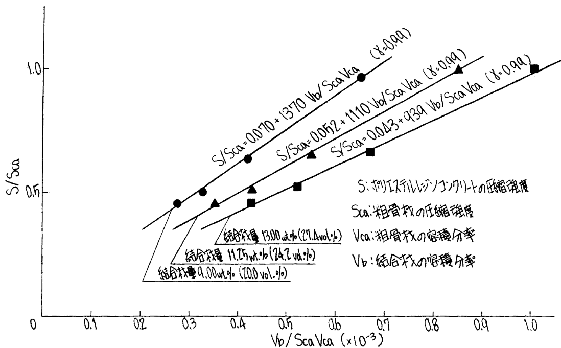
図-3 各結合材量における Vb/ScaVca と S/Sca の関係
