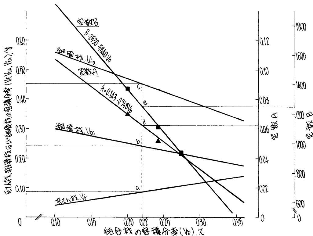
図-4 ポリエステルレジンコンクリートの材料の容積分率の計算図
