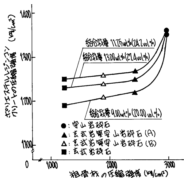
図-1 粗骨材の圧縮強度とポリエステルレジンコンクリートの圧縮強度との関係
