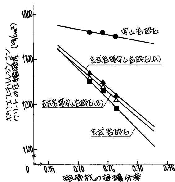
図-2 粗骨材の容積分率とポリエステルレジンコンクリートの圧縮強度との関係
