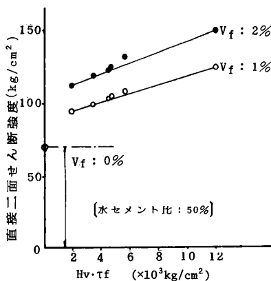
図-10 H_v \cdot \tau_f とせん断強度との関係
