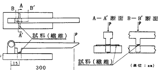
図-2 繊維のせん断強度試験方法
