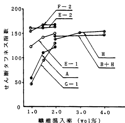
図-14 繊維種類がせん断タフネス指数に及ぼす影響
