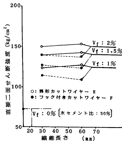
図-6 繊維長さとせん断強度との関係
