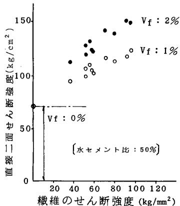
図-9 繊維のせん断強度とせん断強度との関係
