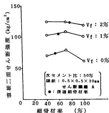
図-4 細骨材率とせん断強度との関係
