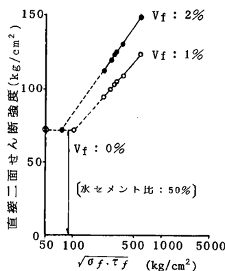
図-11 \sqrt{\sigma_f \cdot \tau_f} とせん断強度との関係
