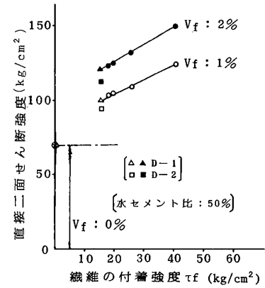
図-7 繊維の付着強度とせん断強度との関係
