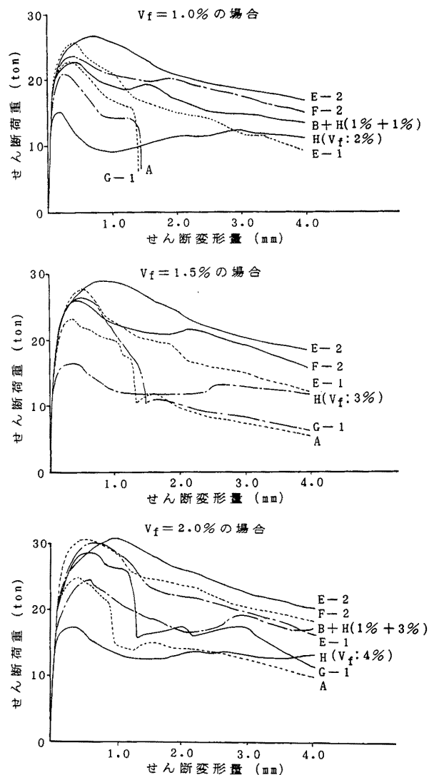
図-13 繊維種類がせん断変形曲線に及ぼす影響
