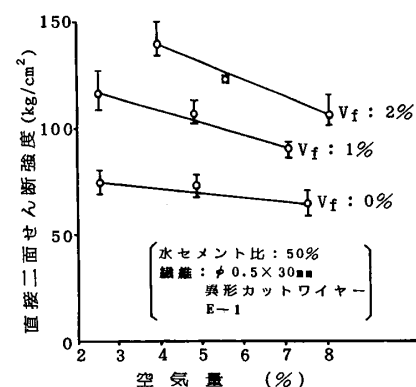
図-5 空気量とせん断強度との関係
