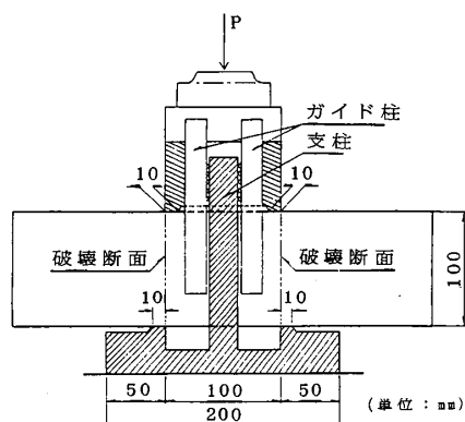
図-1 直接二面せん断強度試験方法
