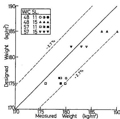
図-2 調合値と測定値の比較 (単位水量)
