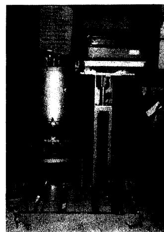
写真-1 調合量測定装置全容
