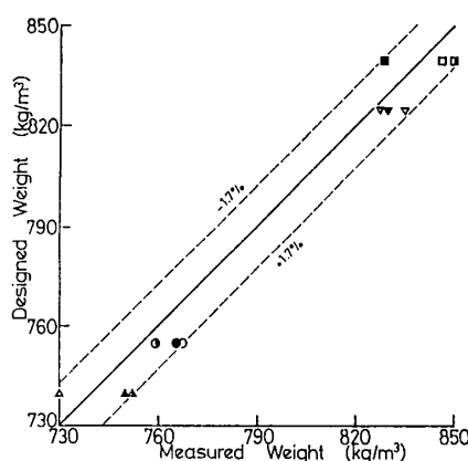
図-4 調合値と測定値の比較 (単位粗骨材量)
