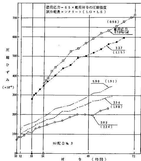
図-3 クリープひずみの試験結果 ( ) 内数値はクリープ係数
