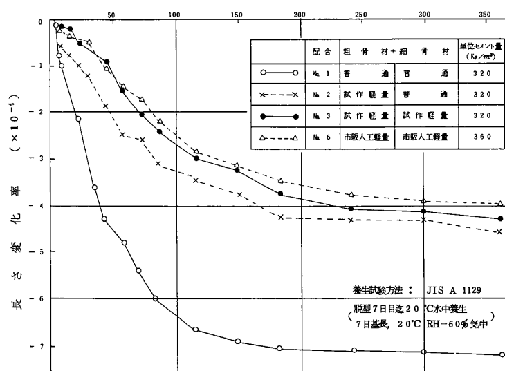
図-4 材令と長さ変化率
