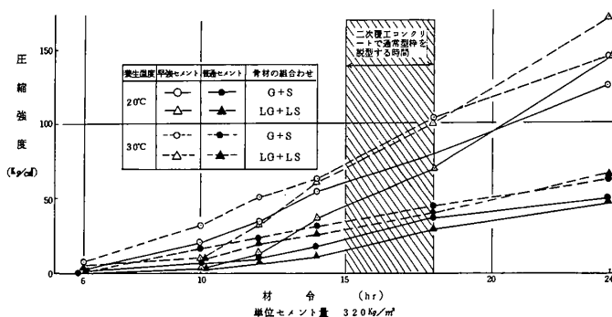
図-2 初期材令における圧縮強度
