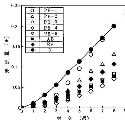
図-4 膨張量と材令の関係（前塗布）
