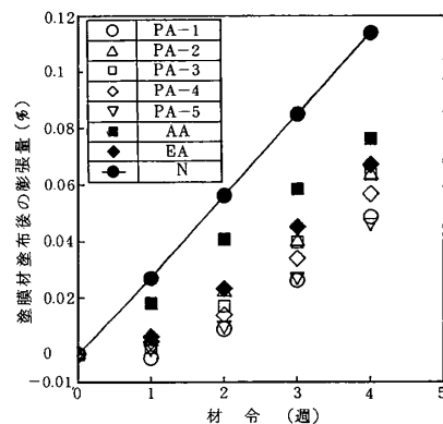
図-5 膨張量と材令の関係（後塗布）
