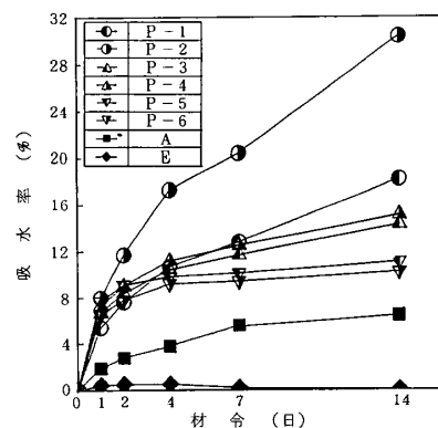
図-3 吸水率試験結果
