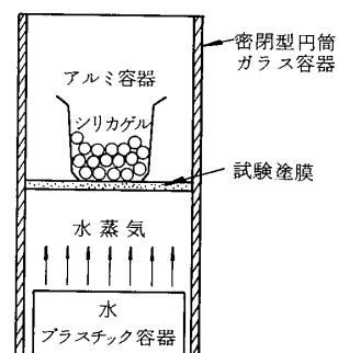
図-1 透湿試験装置
