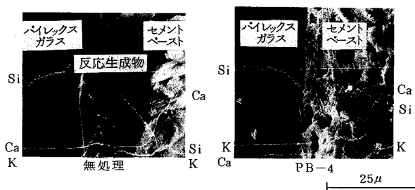
写真-1 パイレックスガラスとセメントペースト界面
