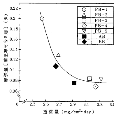
図-6 塗膜材の透湿量と膨張量の関係
