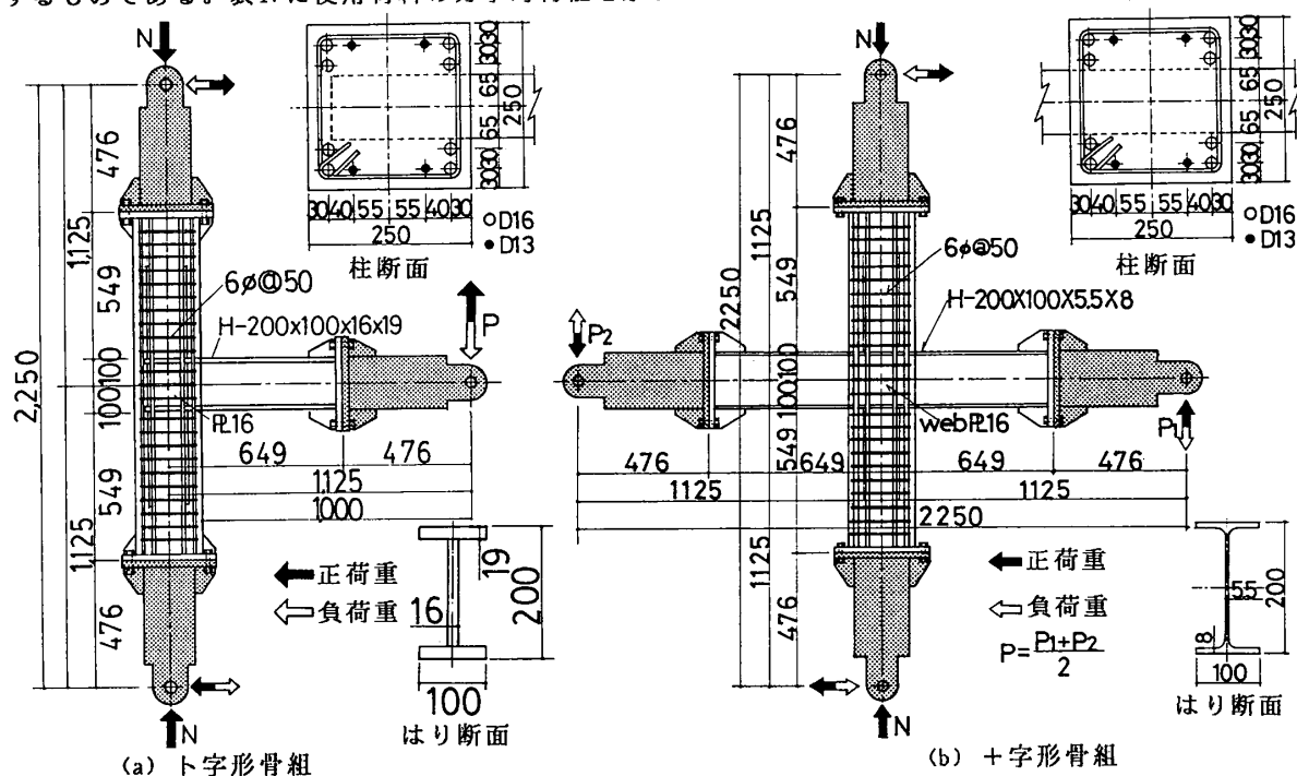
図1. 試験体の形状寸法および断面
