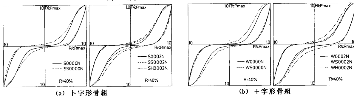
図4. 固有ループ
