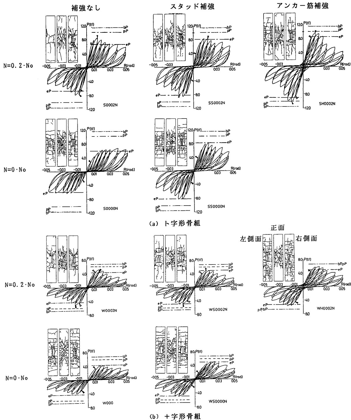
図3. 各試験体の履歴曲線および破壊状況
