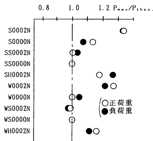
図5. 実験値と解析値との対応
