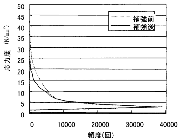
図-12 補強前後の応力頻度分布
