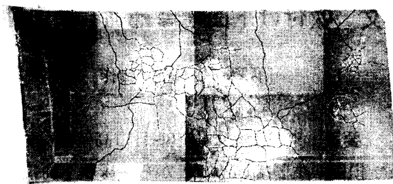
写真-1 床版損傷状況
