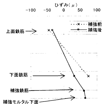
図-5 ひずみ分布
