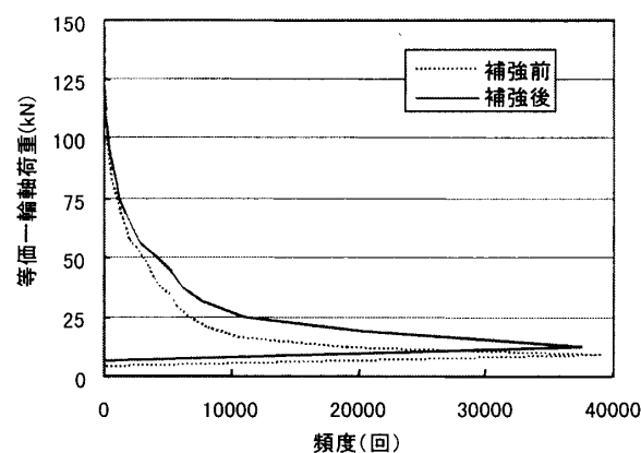
図-13 等価一輪軸荷重と頻度関係
