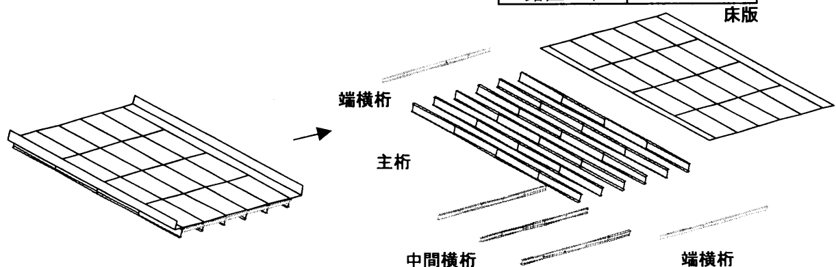
図-4 橋梁解析モデル
