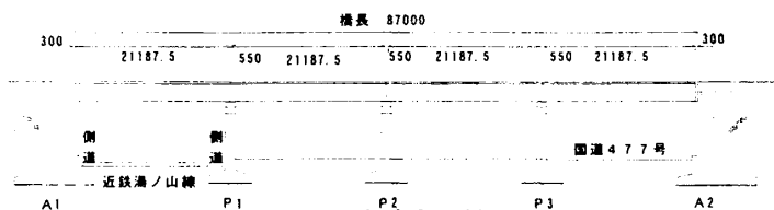
図-1 四日市高架橋概要図
