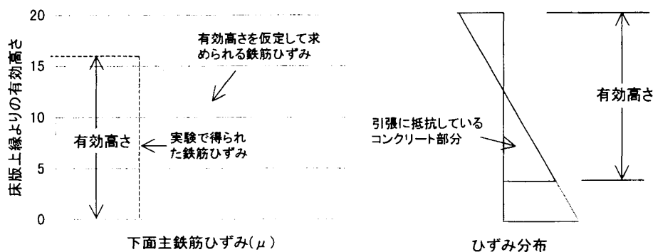
図-11 床版有効高さの仮定
