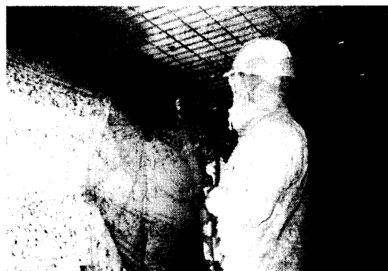
写真-2 吹付け PCM 施工状況 (一層目)
