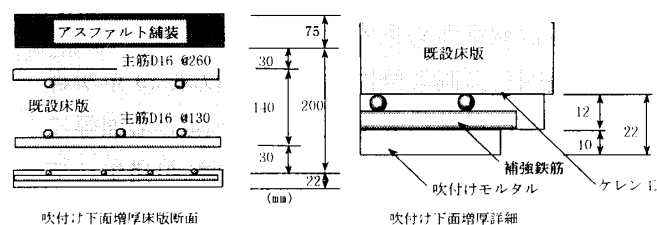
図-2 下面増厚施工断面図
