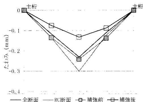
図-7 床版相対たわみ量と計測位置との関係
