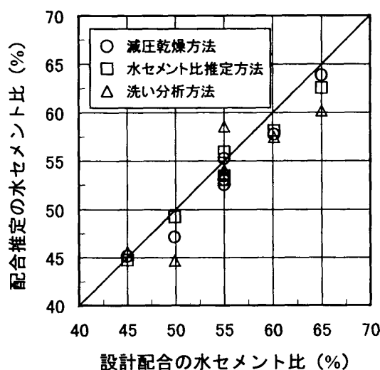
図－６ 設計配合と推定配合の水セメント比
