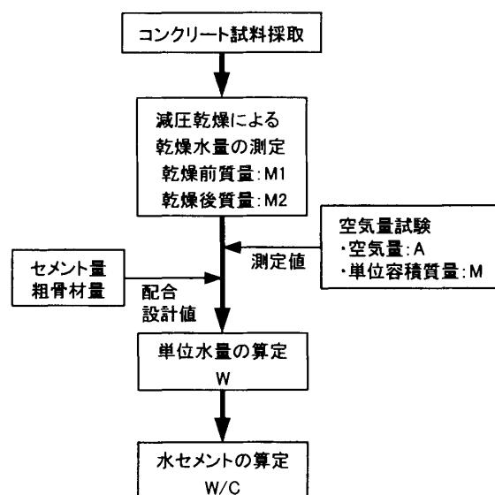
図-2 減圧乾燥方法による算定フロー
