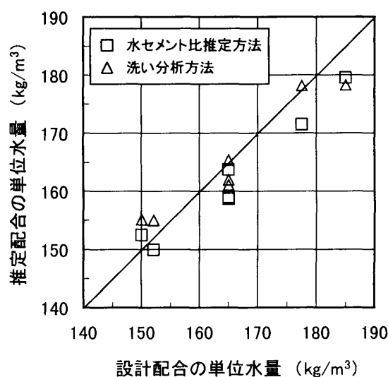
図-5 設計配合と推定配合の単位水量
