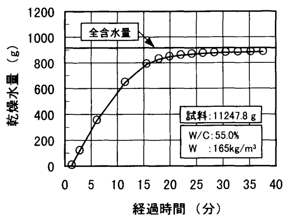
図-3 乾燥水量の時間変化
