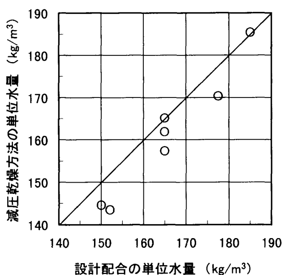
図-4 設計配合と減圧乾燥方法の単位水量
