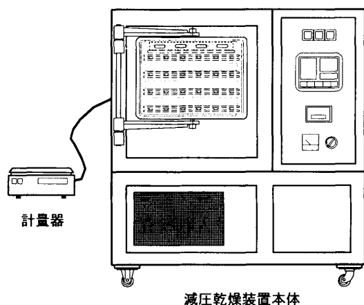
図-1 減圧乾燥装置
