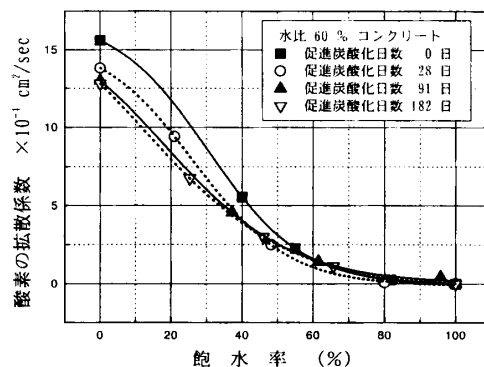
図-6 飽水率と酸素の拡散係数の関係
