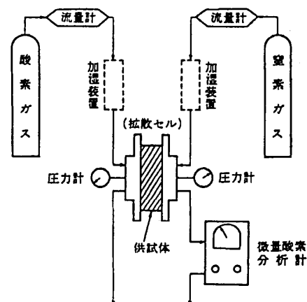
図-5 拡散試験装置の概要
