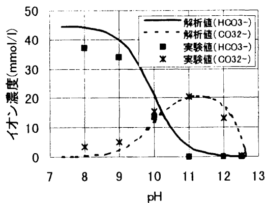
図-4 炭酸イオン及び炭酸水素イオンの変化とpHの関係
