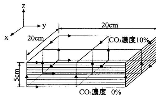
図－３ 解析モデル
