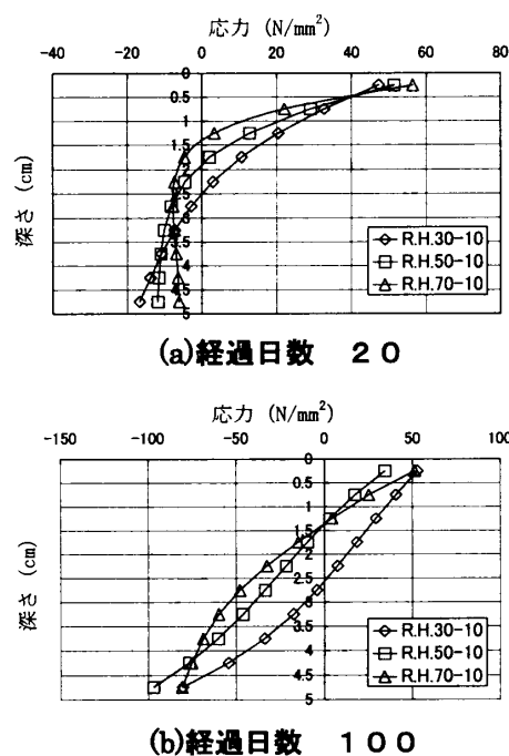
図-5 応力分布 (反応速度定数 1.0)
