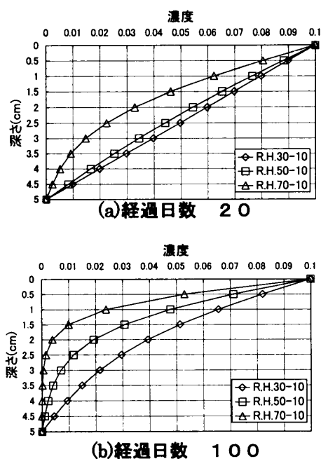
図-4 濃度分布 (反応速度定数 1.0)
