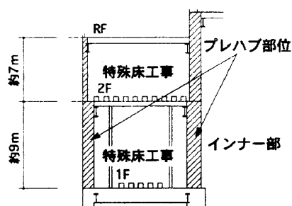
図-4 中央制御室プレハブ位置図
