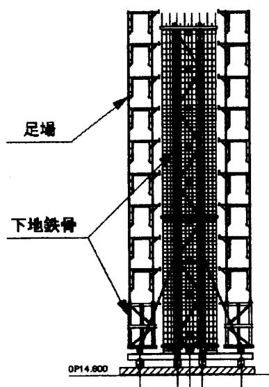
図-7 プレハブ筋組立状況
