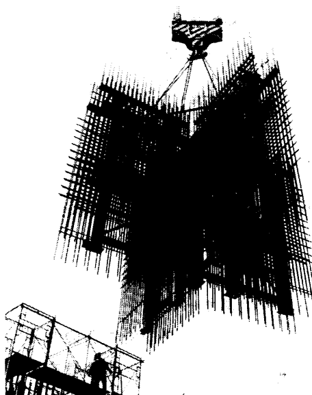
写真-2 十字プレハブ筋吊り込み状況
