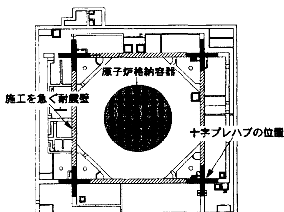
図-3 耐震壁プレハブ位置図
