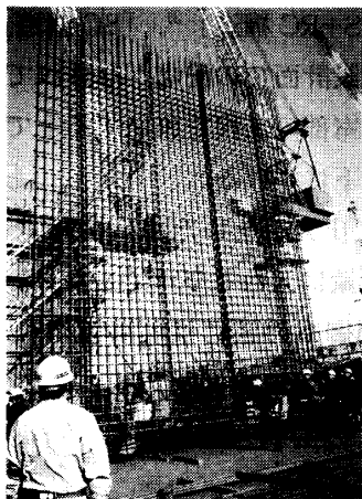
写真-3 壁筋プレハブ吊込み状況
