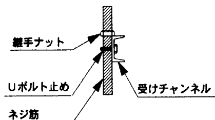
図-6 主筋固定方法詳細図
