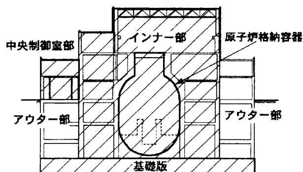
図-2 原子炉建屋断面図
