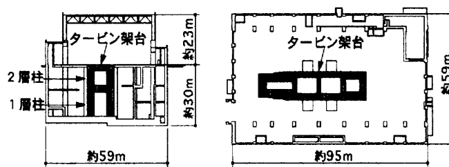
図-5 タービン建屋断面、平面図
