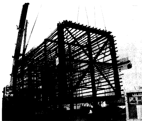
写真-5 2層柱プレハブ筋吊込み状況
