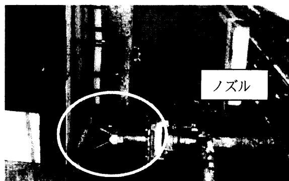
写真-1 接合面処理状況
