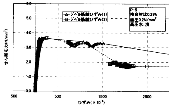
図-4 せん断応力-ひずみ関係
