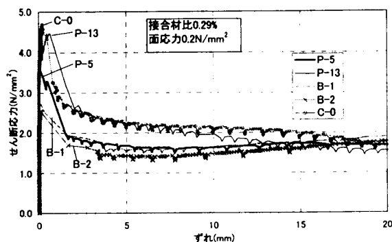
図－3 せん断応力－ずれ関係
