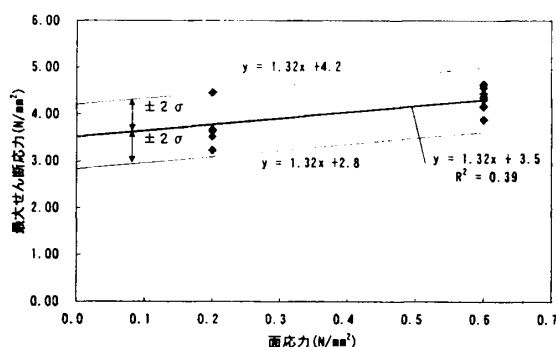
図-7 最大せん断応力回帰直線
