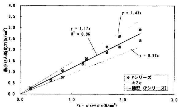
図-8 最小せん断応力回帰直線
