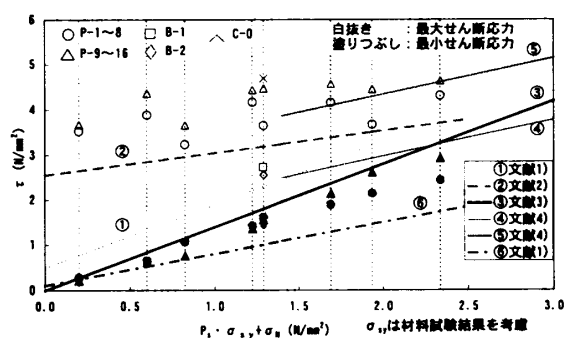
図-6 既往の式と実験結果との比較
