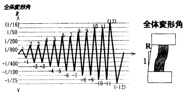
図-7 加力履歴
