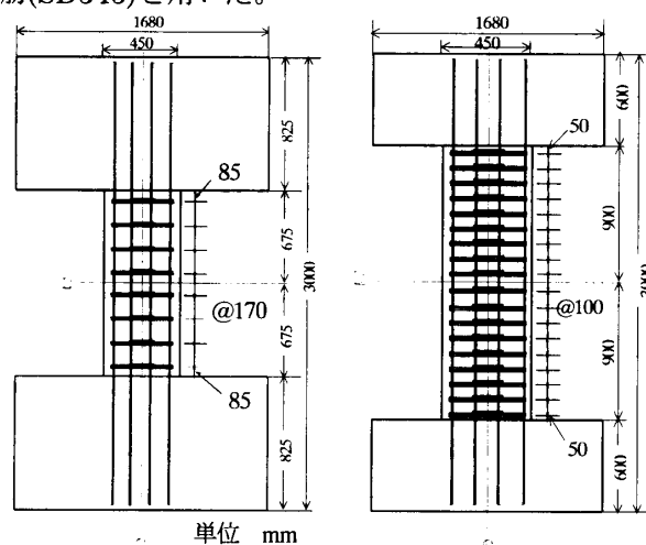
(a) せん断破壊型 (b) 曲げ破壊型
