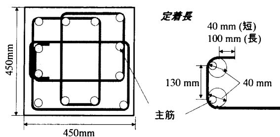
図-5 柱断面
