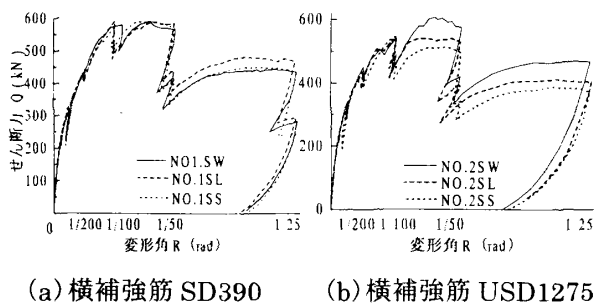
図-10 包絡線による比較（せん断破壊型）
