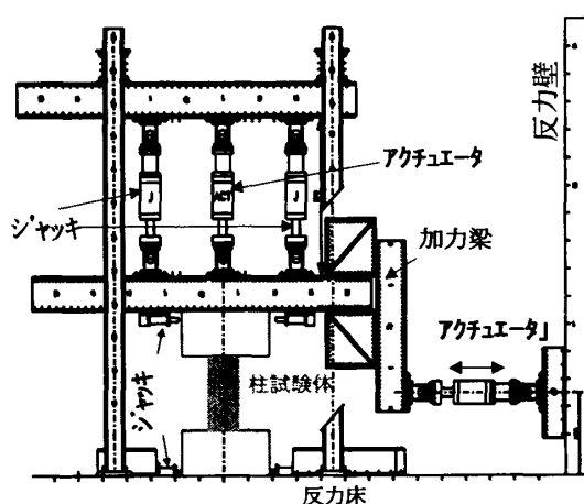
図-6 加力装置
