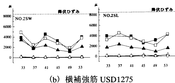
図-13 中段部横補強筋中央のひずみ分布
