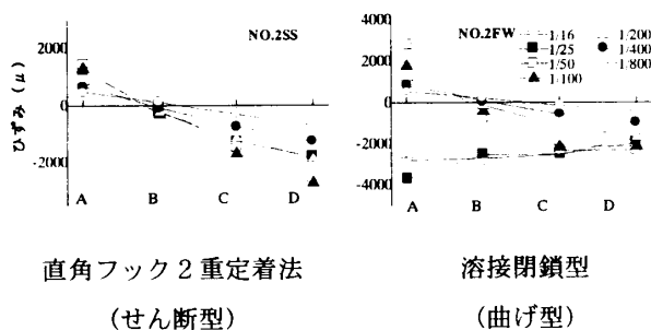
図-12 主筋の柱脚断面のひずみ分布
