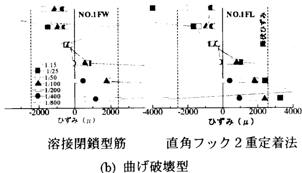
図-11 主筋のひずみ分布 (主筋①)
