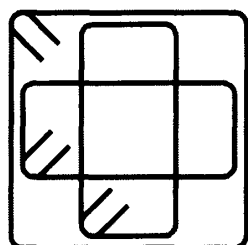
図-1 135^\circ フック定着
