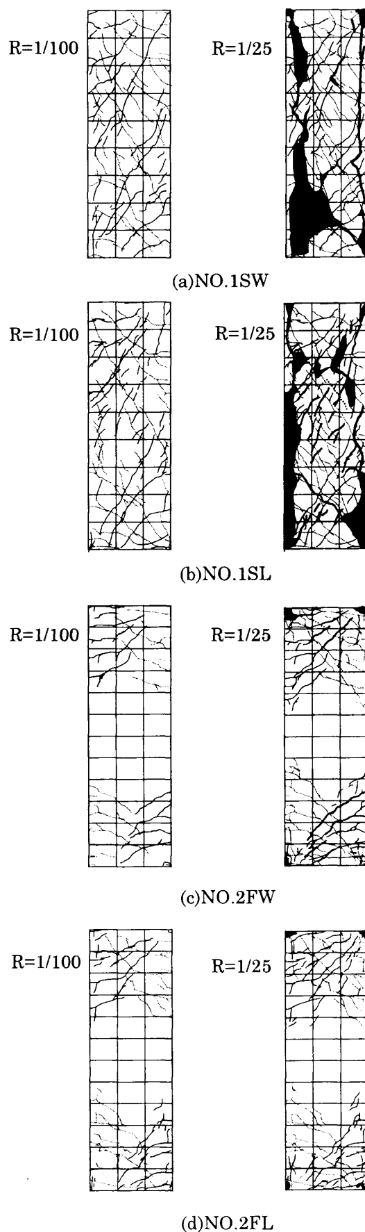
図-8 ひび割れ状況
