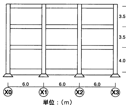
図-1 3層3スパン建物の立面図
