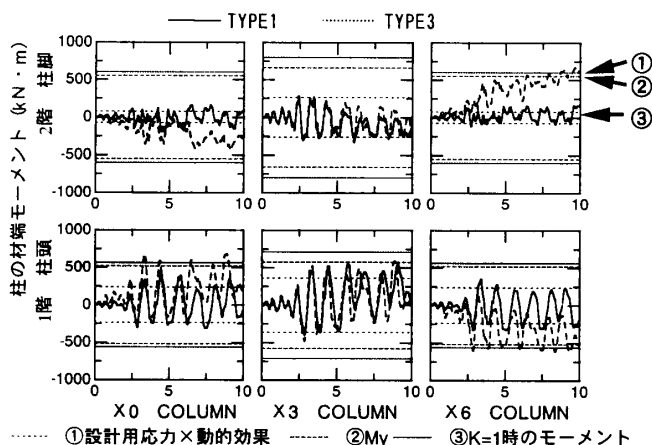
図-1 1 6スパン建物の柱材端モーメント
