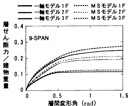
図-7 層せん断力係数-層間変形角関係
