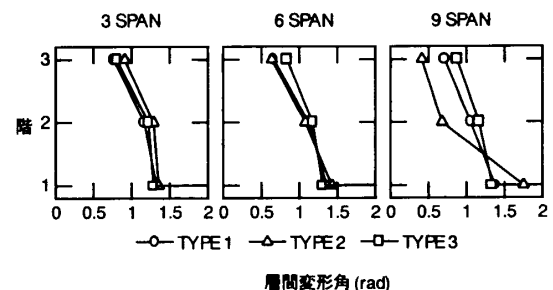
図-10 各階の層間変形角
