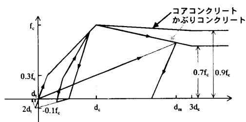
図-5 コンクリートバネの復元力特性
