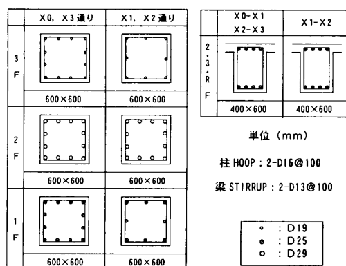
図-2 柱, 梁断面図
