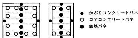
図-4 MSバネへの分割
