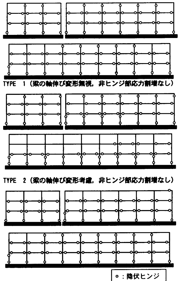
図-9 ヒンジ発生状況
