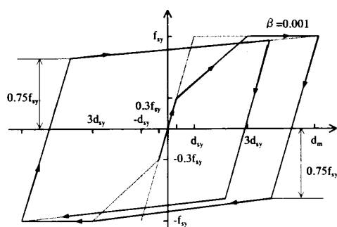
図-6 鉄筋バネの復元力特性
