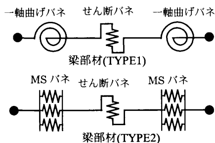
図-3 梁部材のモデル化
