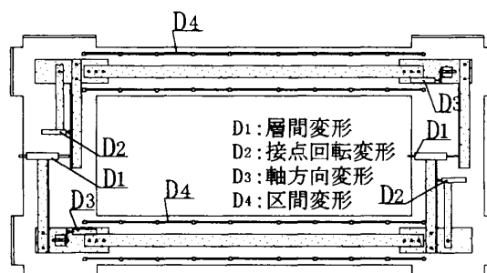
図-2 変形等の測定方法
