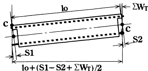
(b) SL-FRAME の場合
