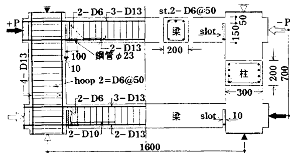
図-1 試験体(SL-FRAME)の形状、寸法、配筋等
