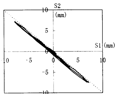
図-12 SL-FRAME 梁端下端筋位置の区間変形
