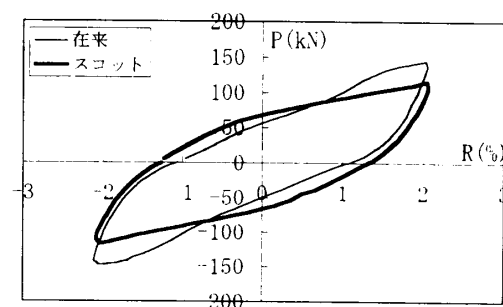
(b) R=2% 時のループの形状
