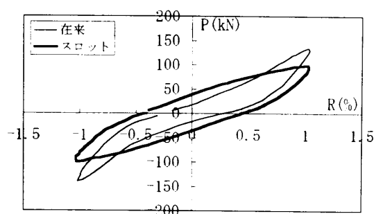
(a) R=1% 時のループの形状
