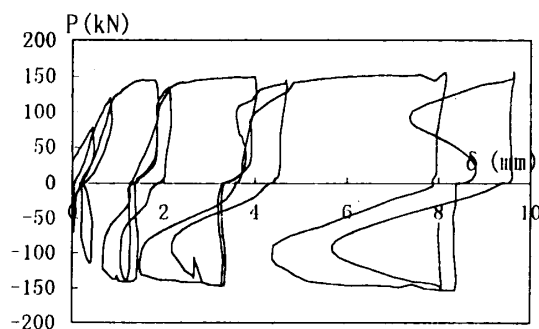
(a)上梁の軸方向変形挙動
