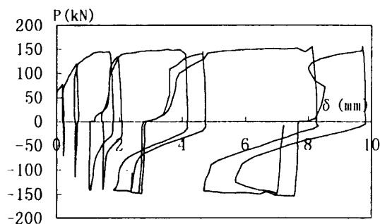
(b)下梁の軸方向変形挙動
