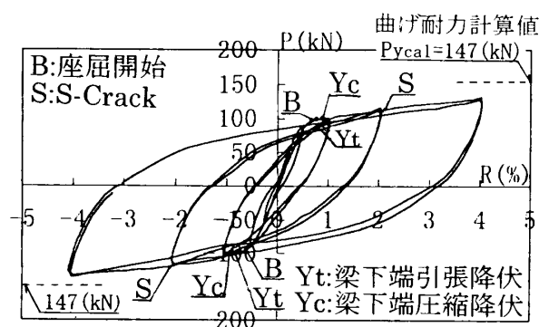
図-3 SL-FRAME の荷重変形曲線
