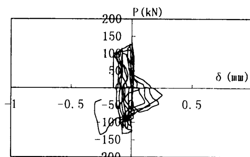
(b)下梁の軸方向変形挙動
