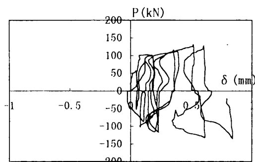
(a)上梁の軸方向変形挙動
