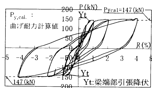
図-4 RC-FRAME の荷重変形曲線
