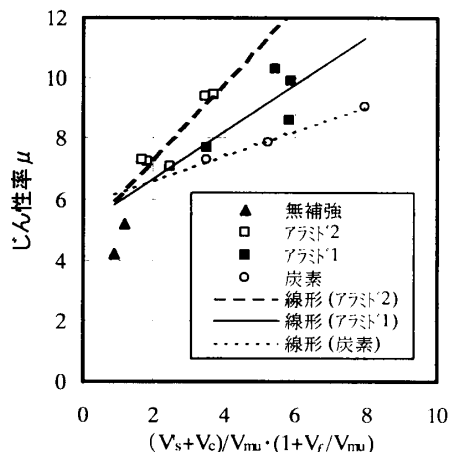
図-7 (V'_s+V_c)/V_{mu} \cdot (1+V_f/V_{mu}) とじん性率の関係
