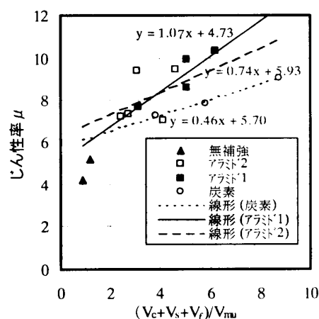
図-1 せん断余裕度とじん性率の関係
