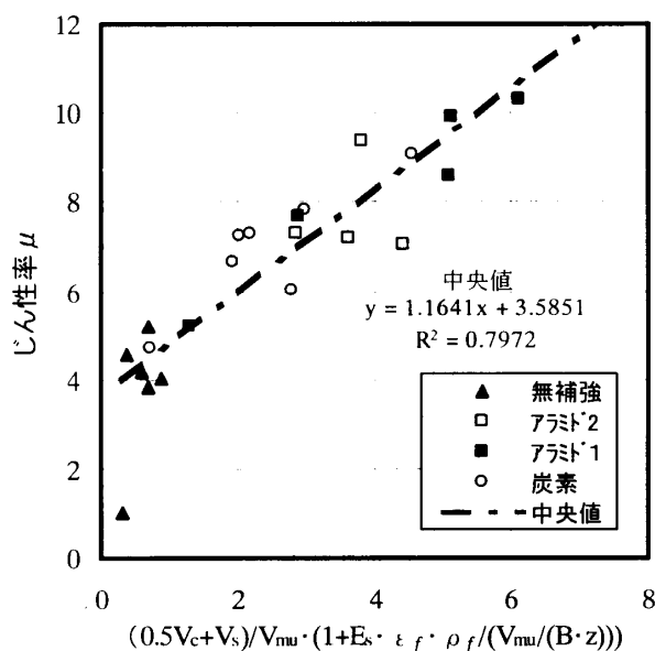
図-10 じん性率評価（実験値）
