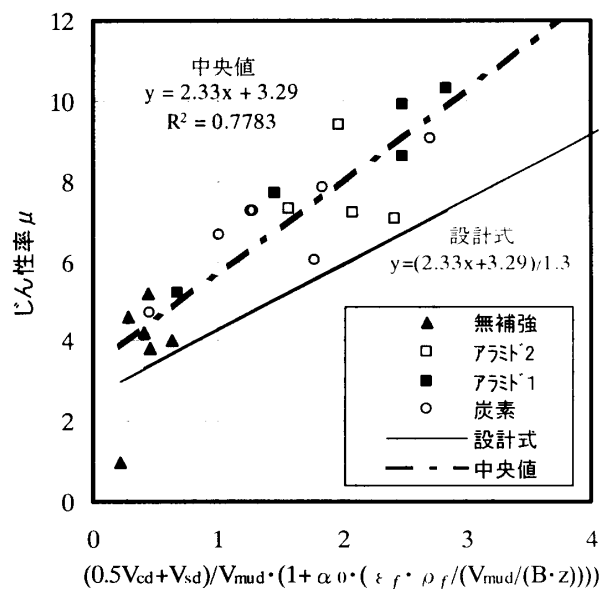
図-11 じん性率評価（設計値使用）
