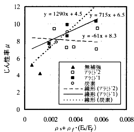
図-4 せん断補強量とじん性率の関係
