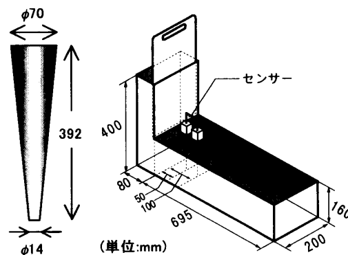
図-1 J 14 漏斗, L フロー試験器
