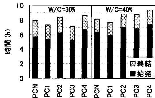
図-11 凝結時間
