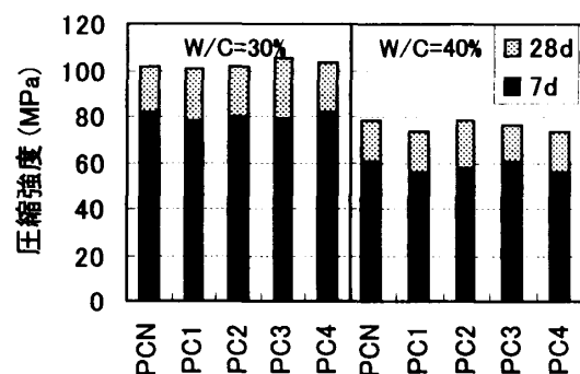
図-12 圧縮強度
