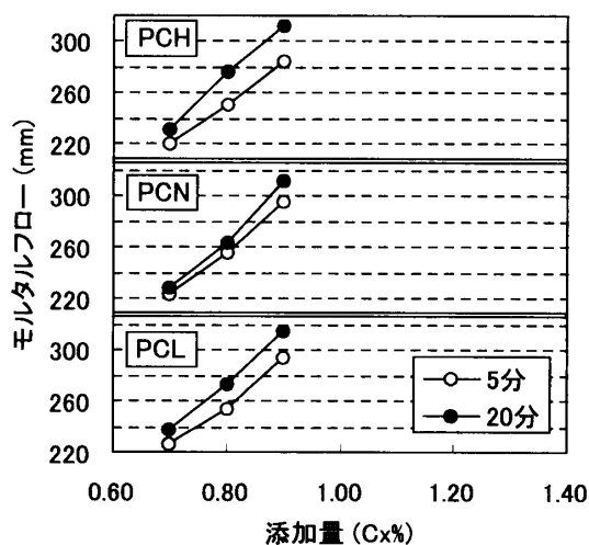
図-5 PC 添加量とモルタルフロー
