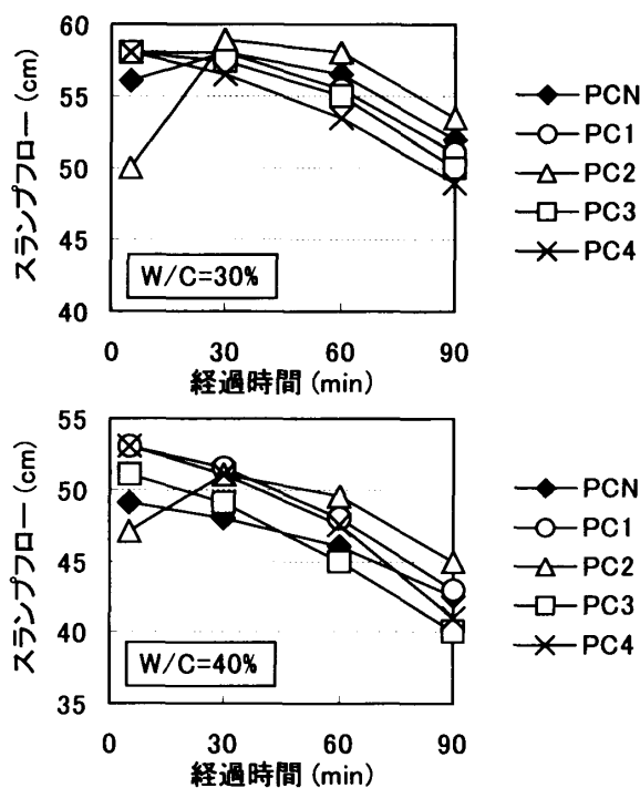
図-8 スランプフローの経時変化
