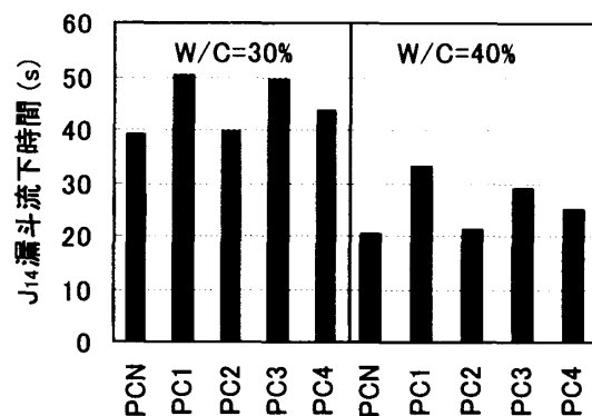
図-10 J_{14} 漏斗流下時間
