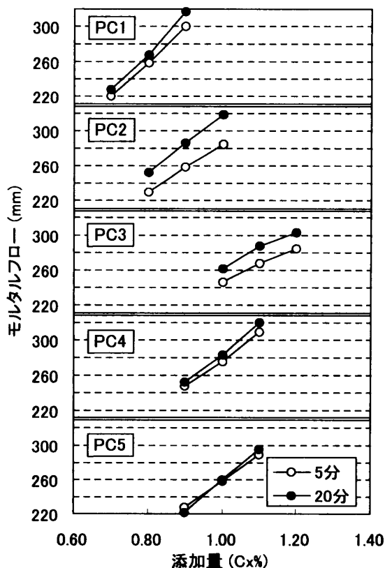
図-2 PC 添加量とモルタルフロー
