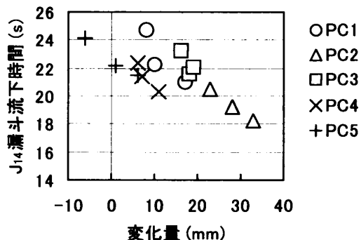
図-4 練混ぜ後 5 分から 20 分のフローの差と粘性
