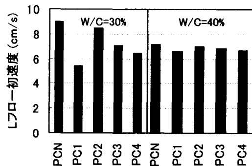
図-9 Lフロー初速度
