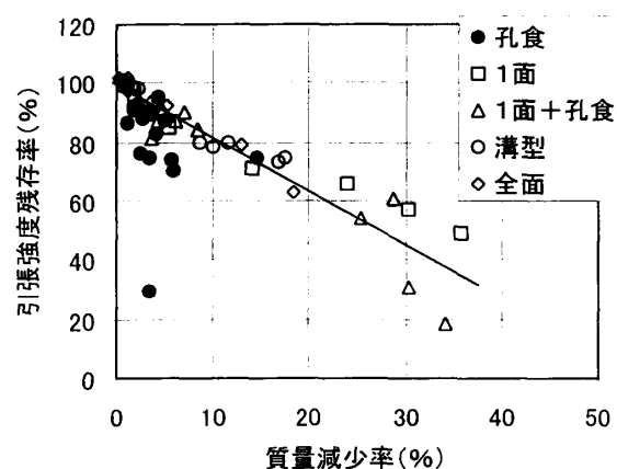
図-6 質量減少率と引張強度残存率の関係
