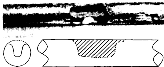
写真-1 著しい孔食の例
