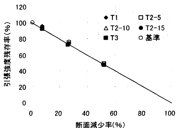
注) 図中には同一タイプ3本の 平均値をプロットした。 図-10 断面減少率と引張強度残存率の関係
