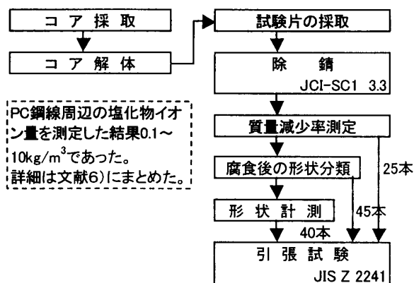
図-1 シリーズ1の実験概要
