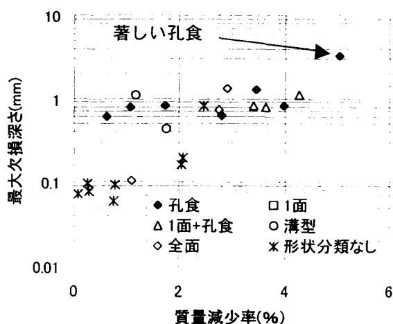
図-4 質量減少率と最大欠損深さの関係
