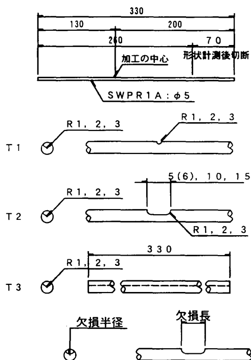
図-3 試験片形状 (シリーズ2)
