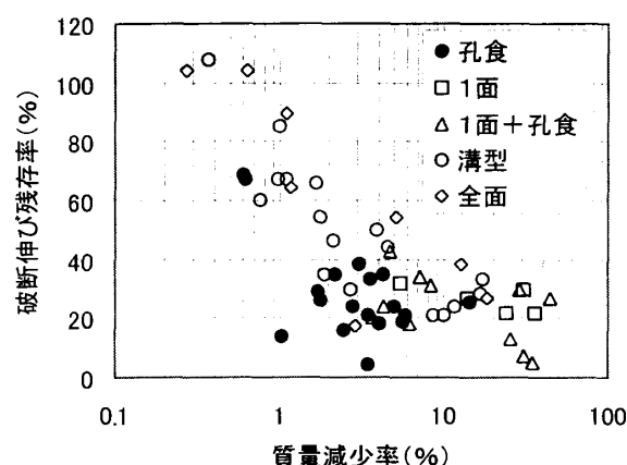
図-7 質量減少率と破断伸び残存率の関係
