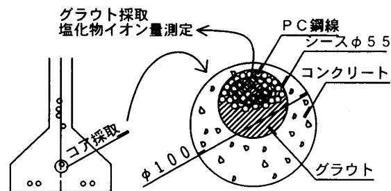
図-2 試験片の採取概要図
