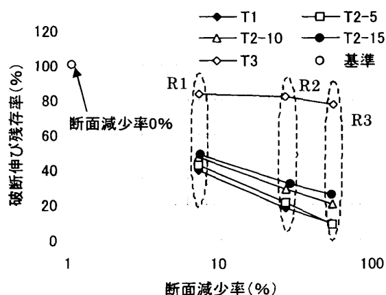
注) 図中には同一タイプ3本の 平均値をプロットした。 図-11 断面減少率と破断伸び残存率の関係
