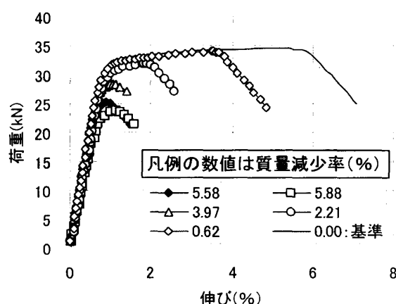
図-5 荷重伸び曲線（シリーズ1：孔食）
