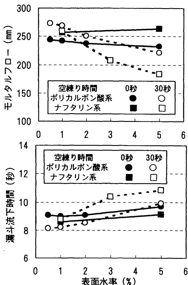
図-8 表面水率と初期流動特性の関係
