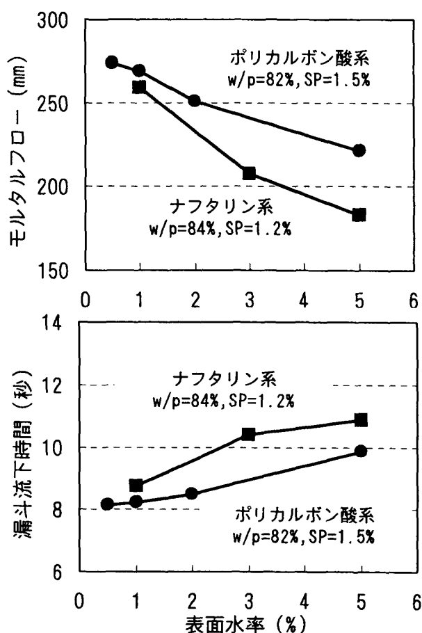
図-2 表面水率と初期流動特性の関係
