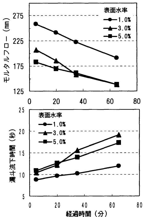
図-4 流動特性の経時変化 (ナフタリン系)
