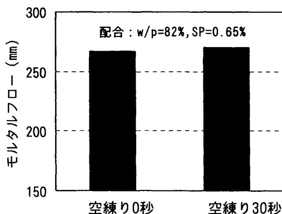
図-6 モルタルフローと空練り時間 (石灰石微粉末単味)
