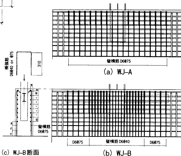
図-8 耐震壁配筋
