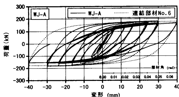
図-10 荷重変形関係
