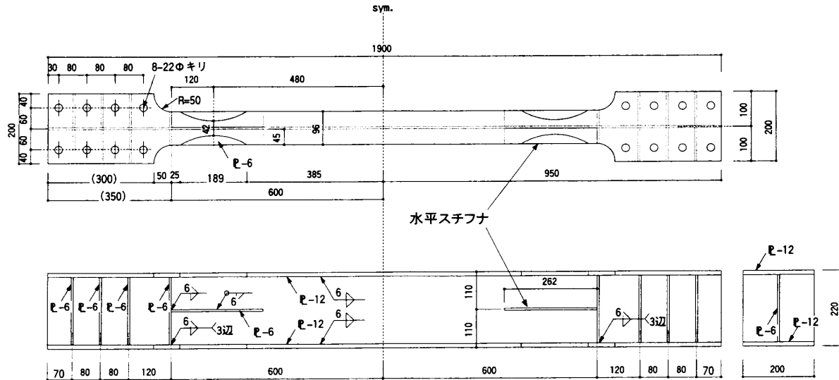
図-2 No.6 試験体概要図
