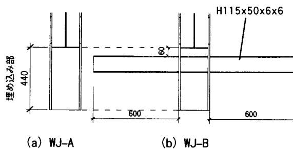
図-7 連結部材埋め込み部
