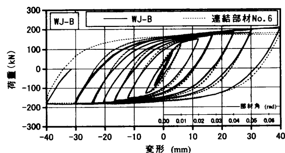
図-10 荷重変形関係
