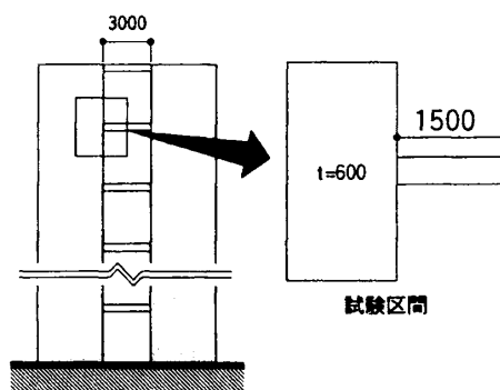
図-5 接合部実験の検討対象範囲
