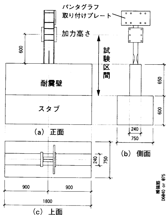
図-6 試験体概観(WJ-A,B 共通)
