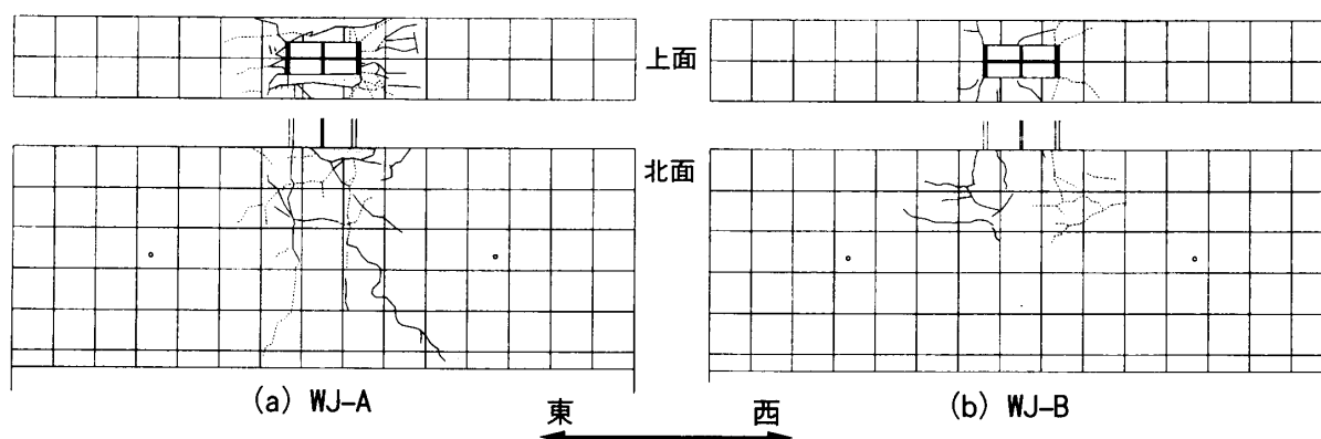
図-11 実験終了時ひび割れ図
