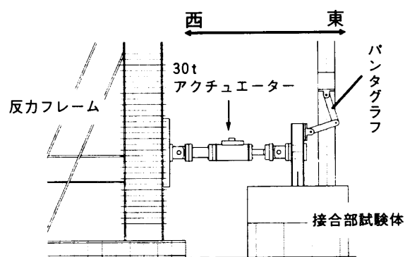
図-9 加力装置図
