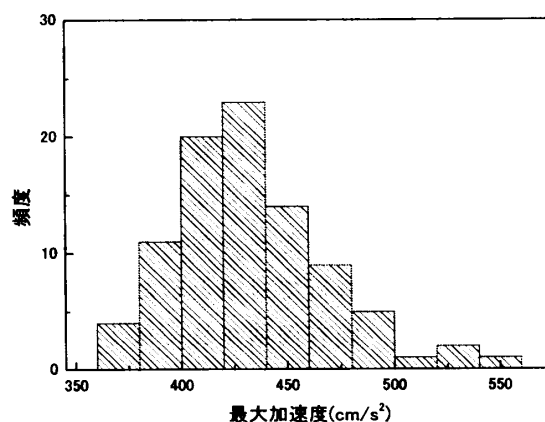
図-5 最大加速度分布
