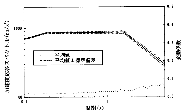
図-3 加速度応答スペクトル
