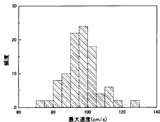
図-6 最大速度分布
