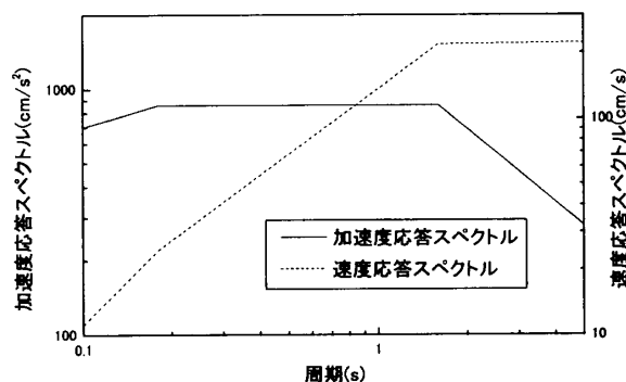
図-1 道路橋示方書設計スペクトル
