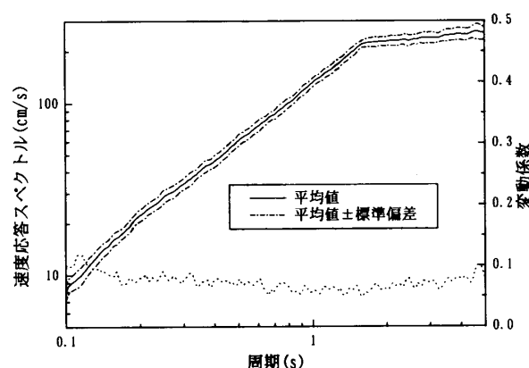
図-4 速度応答スペクトル
