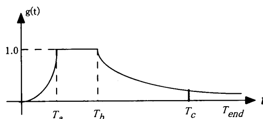
図-2 Jennings型包絡関数
