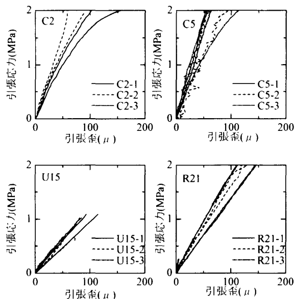
図-3 P-Test 応力-歪（ゲージ）関係
