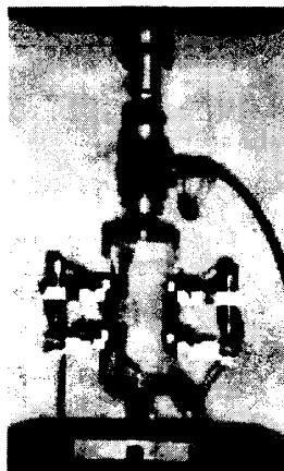
図-6 試験体設置状況
