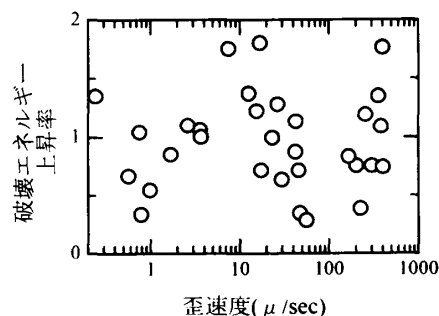
図－11 破壊エネルギー上昇率－歪速度関係
