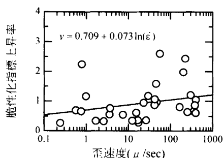
図-12 脆性化指標上昇率-歪速度関係
