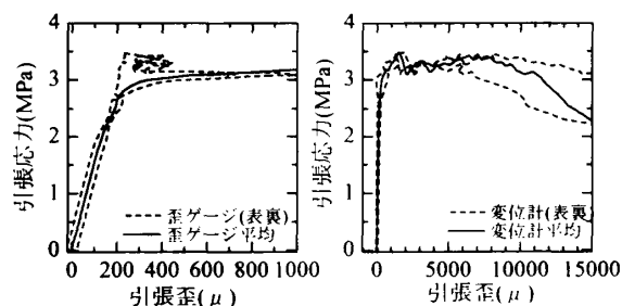
図-5 P-Test 応力-歪関係
