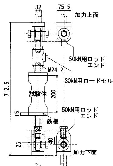
図-2 P-PTest 試験体
