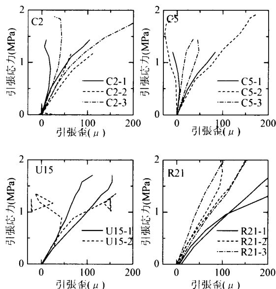
図-1 BRI-GripTest 応力-歪 (ゲージ) 関係
