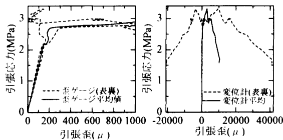
図-4 P-Test 応力-歪関係
