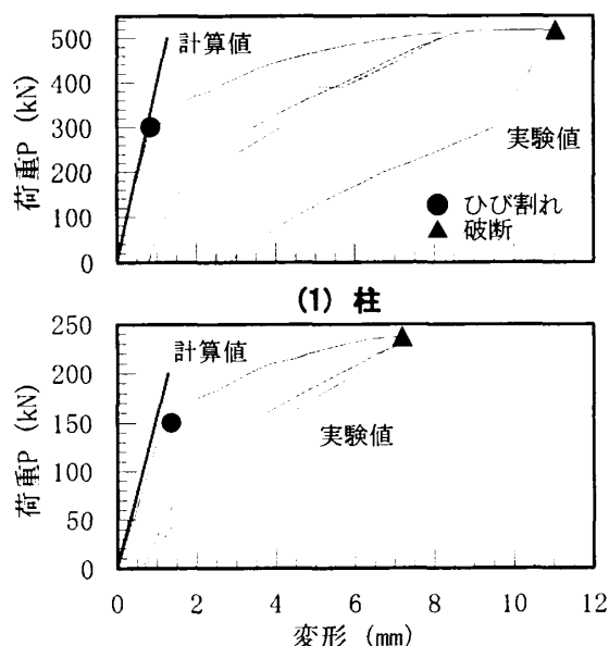
図-4 荷重-変形関係 (柱及び梁の曲げ実験)
