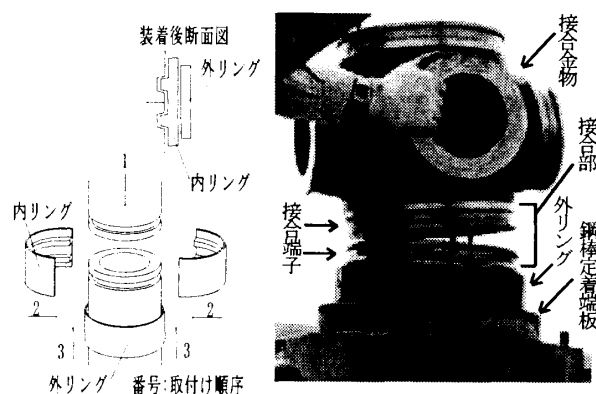
図-2 部材接合部
