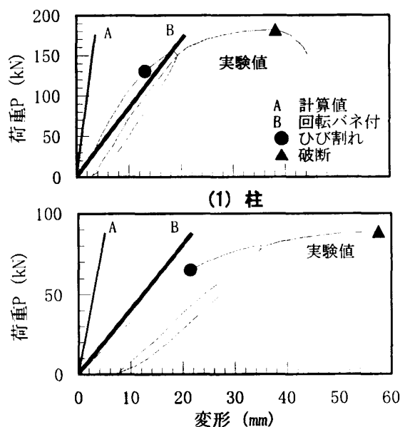
図-6 荷重-変形関係 (接合部の曲げ実験)
