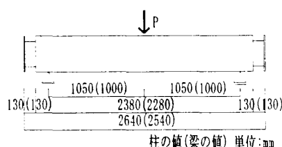
図-3 柱及び梁の曲げ実験
