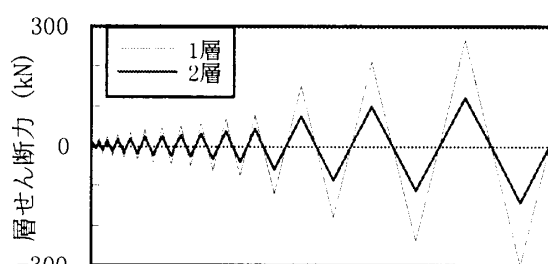
図-9 荷重履歴
