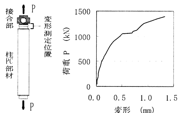
図-7 接合部の引張実験
