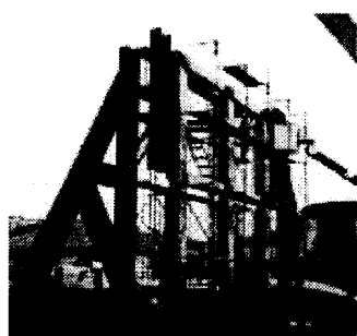
写真-3 載荷装置と実験用ラーメン
