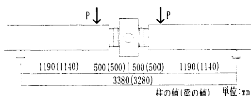
図-5 接合部の曲げ実験
