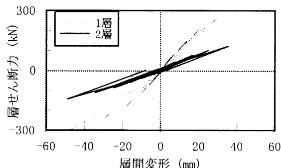
図-10 層せん断力-層間変形関係
