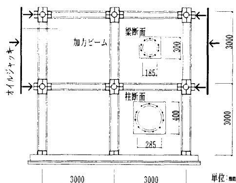
図-1 実験用ラーメンおよび部材断面
