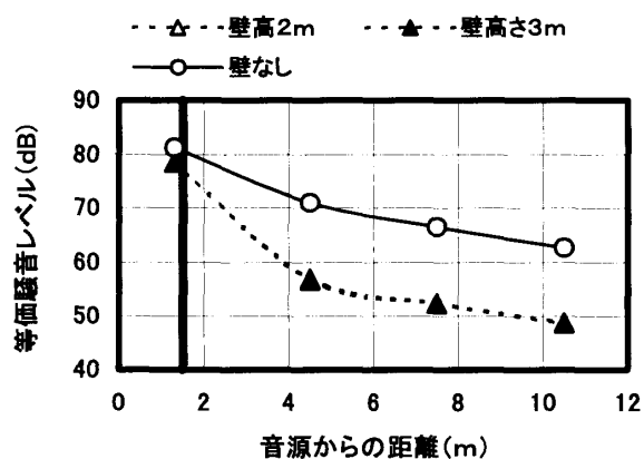
図-7 各受音点での騒音レベル (壁長5m, 受音高2.3m)
