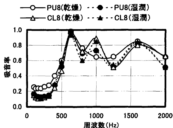
図-3 骨材の種類と乾湿条件が吸音率一周波数間に及ぼす影響
