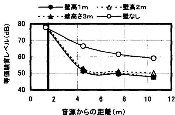
図-10 各受音点での騒音レベル (壁長3m, 受音高さ0.75m)
