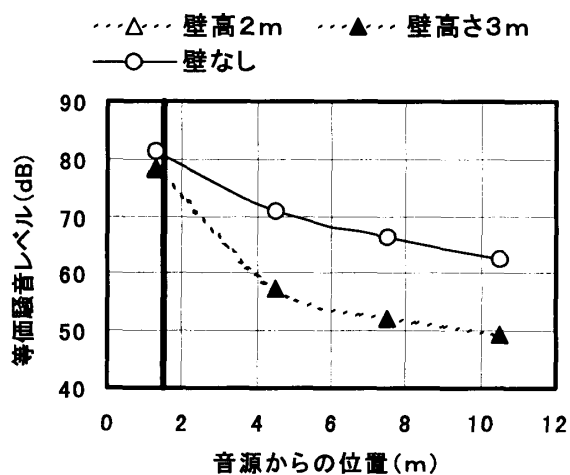
図-9 各受音点での騒音レベル (壁長4m, 受音高2.3m)
