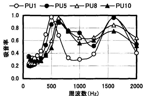
図-1 吸音率一周波数関係 (ぼら)
