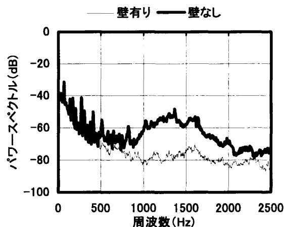
図-5 壁の有無が周波数特性に及ぼす影響（受音点2）
