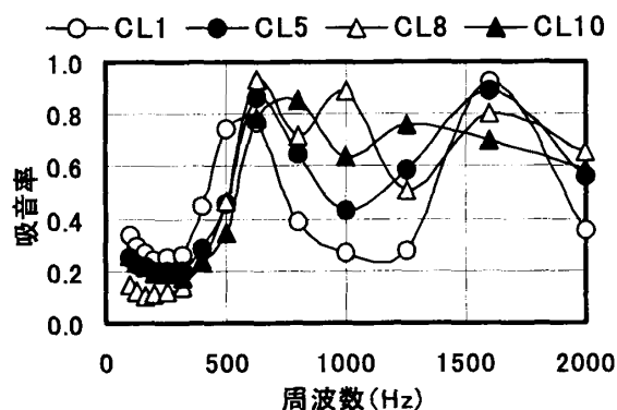
図-2 吸音率一周波数関係 (石灰石)
