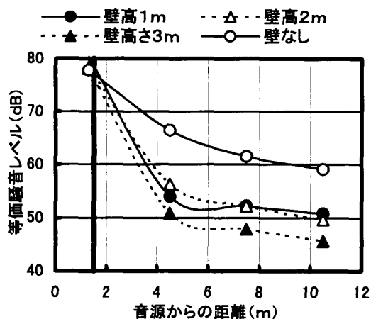
図-6 各受音点での騒音レベル (壁長5m, 受音高0.75m)
