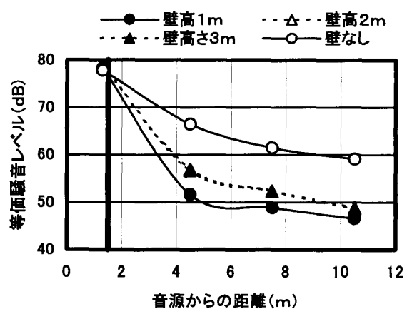
図-8 各受音点での騒音レベル (壁長4m, 受音高0.75m)
