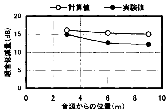
図-13 回折行路差による騒音低減量 (壁高2m, 受音高さ0.75m)
