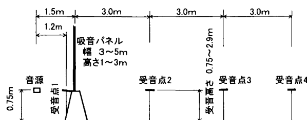
図-4 吸音壁の設置状況と騒音測定位置
