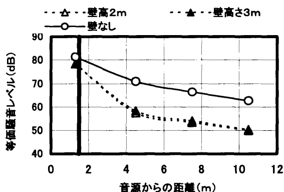
図-11 各受音点での騒音レベル (壁長3m, 受音高さ2.3m)
