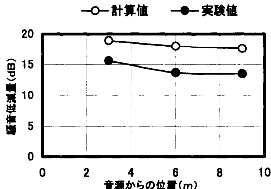
図-14 回折行路差による騒音低減量 (壁高3m, 受音高さ0.75m)
