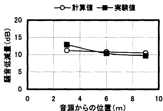
図-12 回折行路差による騒音低減量 (壁高1m, 受音高さ0.75m)
