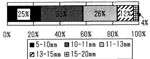
図-2 再生粗骨材の粒度構成
