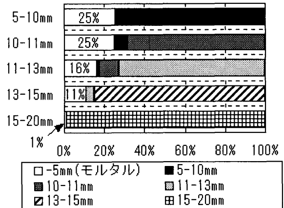
図-2 再生粗骨材の粒度構成
