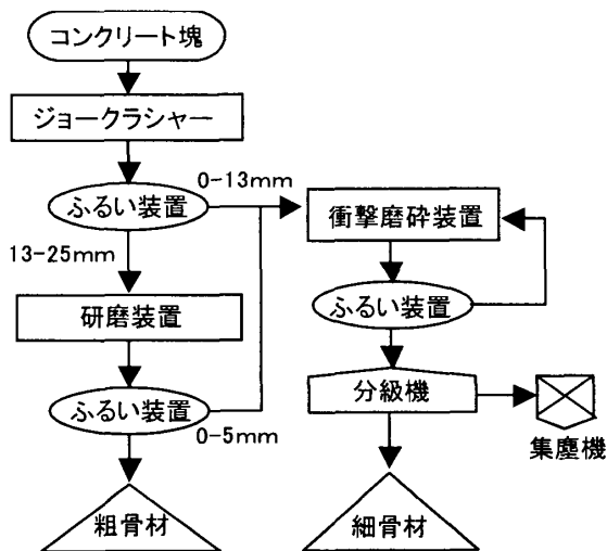
図-1 再生骨材の製造
