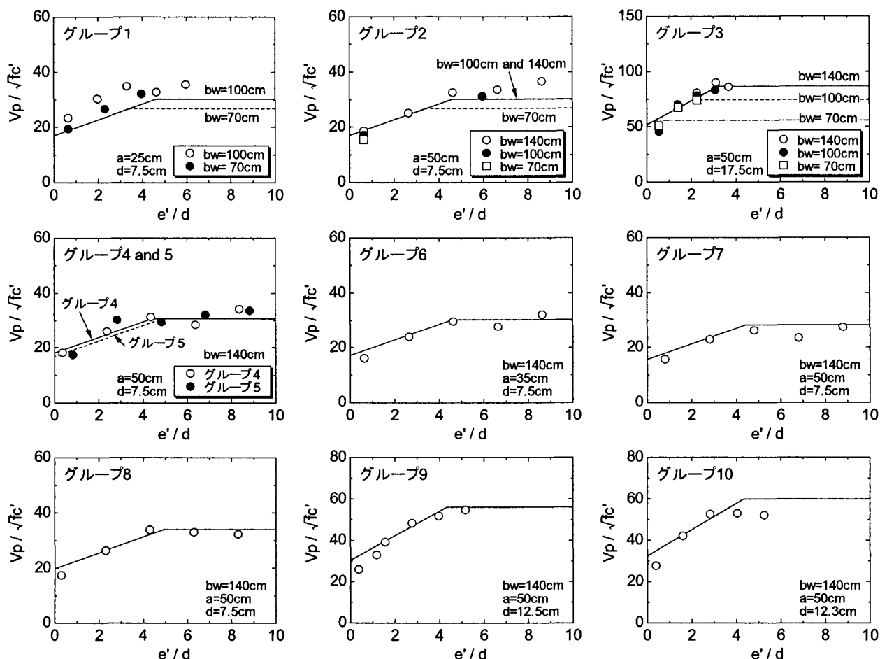
図-9 補正された押抜きせん断耐方式による試算結果
