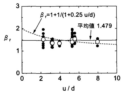
図-8 載荷周長の影響
