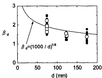
図-6 寸法効果の影響
