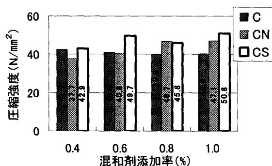
図-10 圧縮強度
