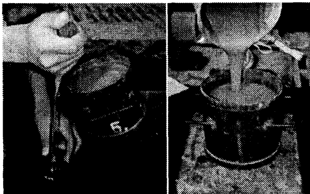
図-3 ブリーディング試験状況
