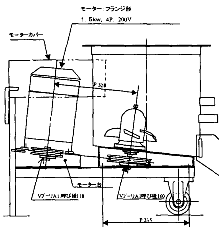
図－１ 新型ミキサの形状
