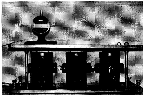
図-4 収縮試験状況
