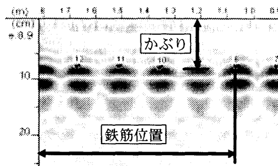
図-2 電磁波レーダ法によって得られた波形データの一例
