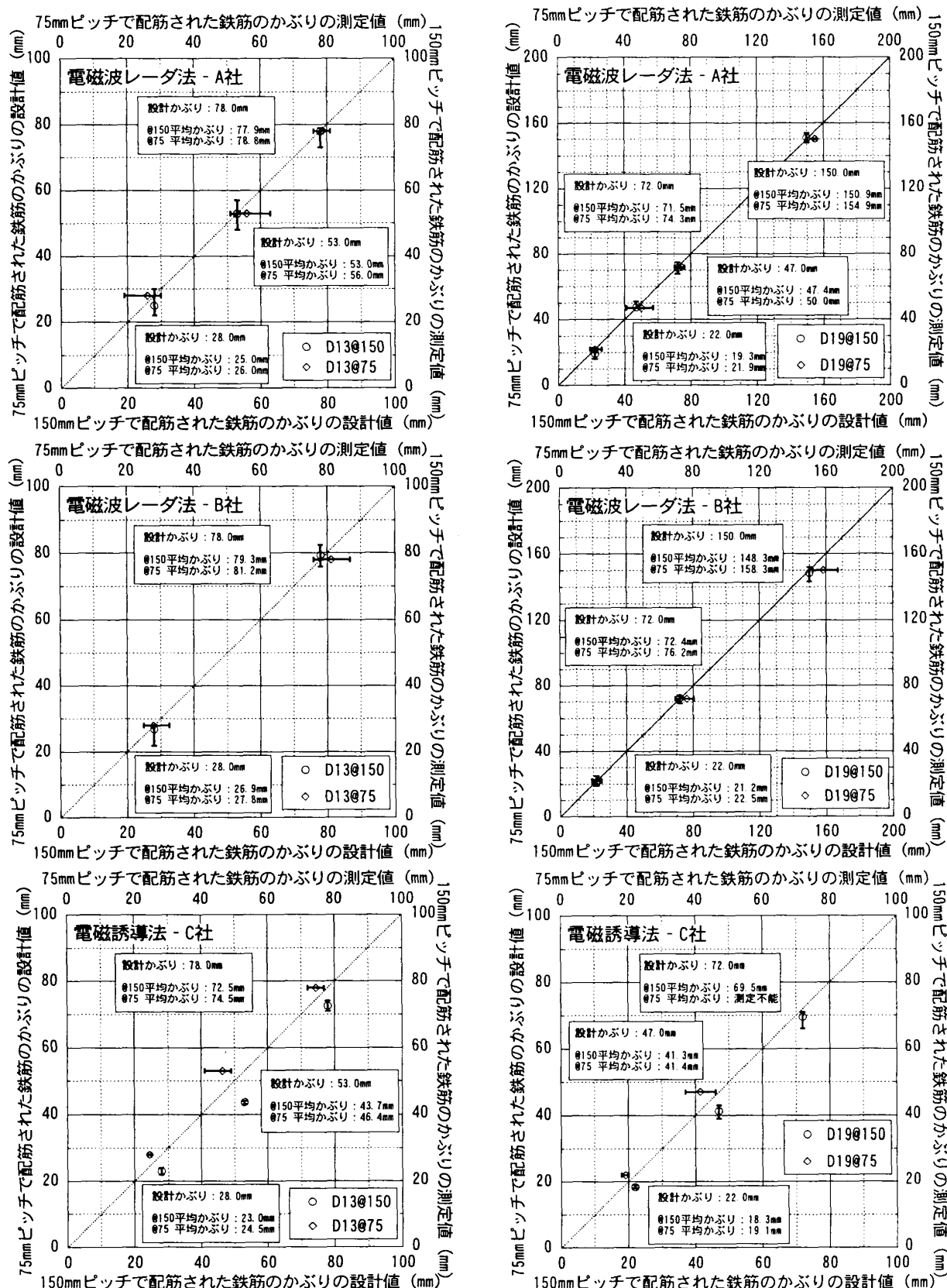
図-4 配筋間隔が異なる同径鉄筋のかぶり測定値の比較
