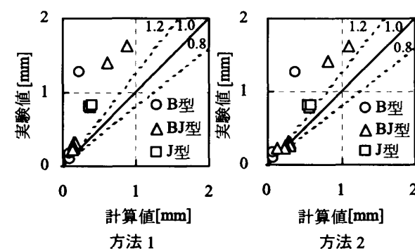
図-8 めり込み量
