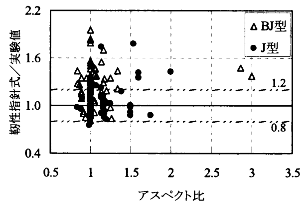
接合部靱性指針式
