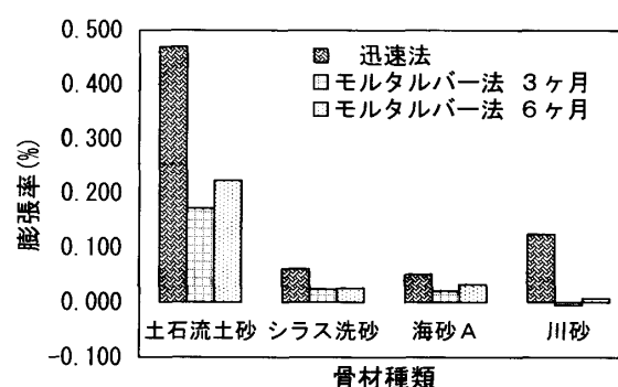
図-2 迅速法とモルタルバー法による膨張率
