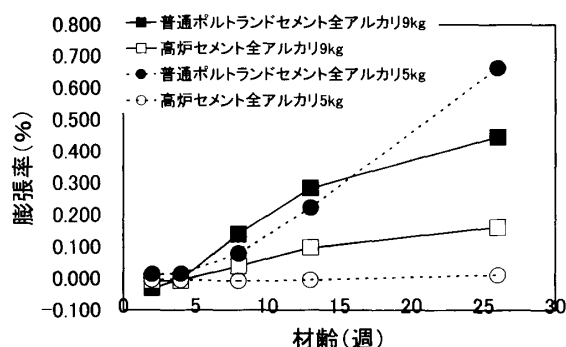
図-5 コンクリートの膨張率
