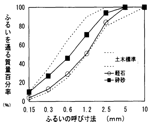
図-6 骨材の粒度曲線
