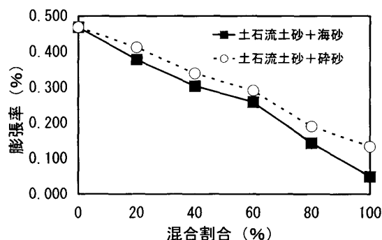
図-3 混合砂のアルカリシリカ反応性
