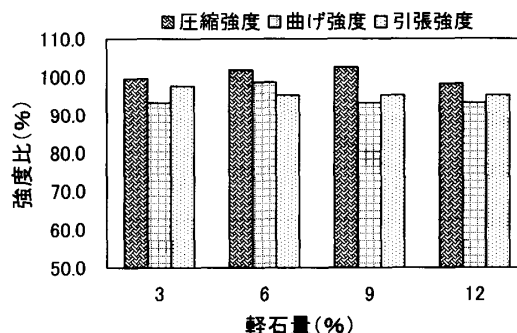
図-8 コンクリートの軽石量と強度比
