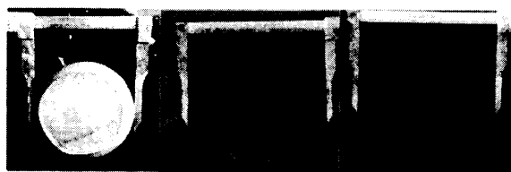
写真-2 スラグ添加型・高粘性型・低粘性型 グラウトのフロー状況
