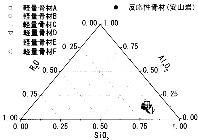
図－2 軽量骨材の化学組成 (SEM-EDX 分析)
