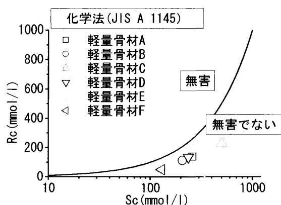
図-3 軽量骨材の化学法の結果
