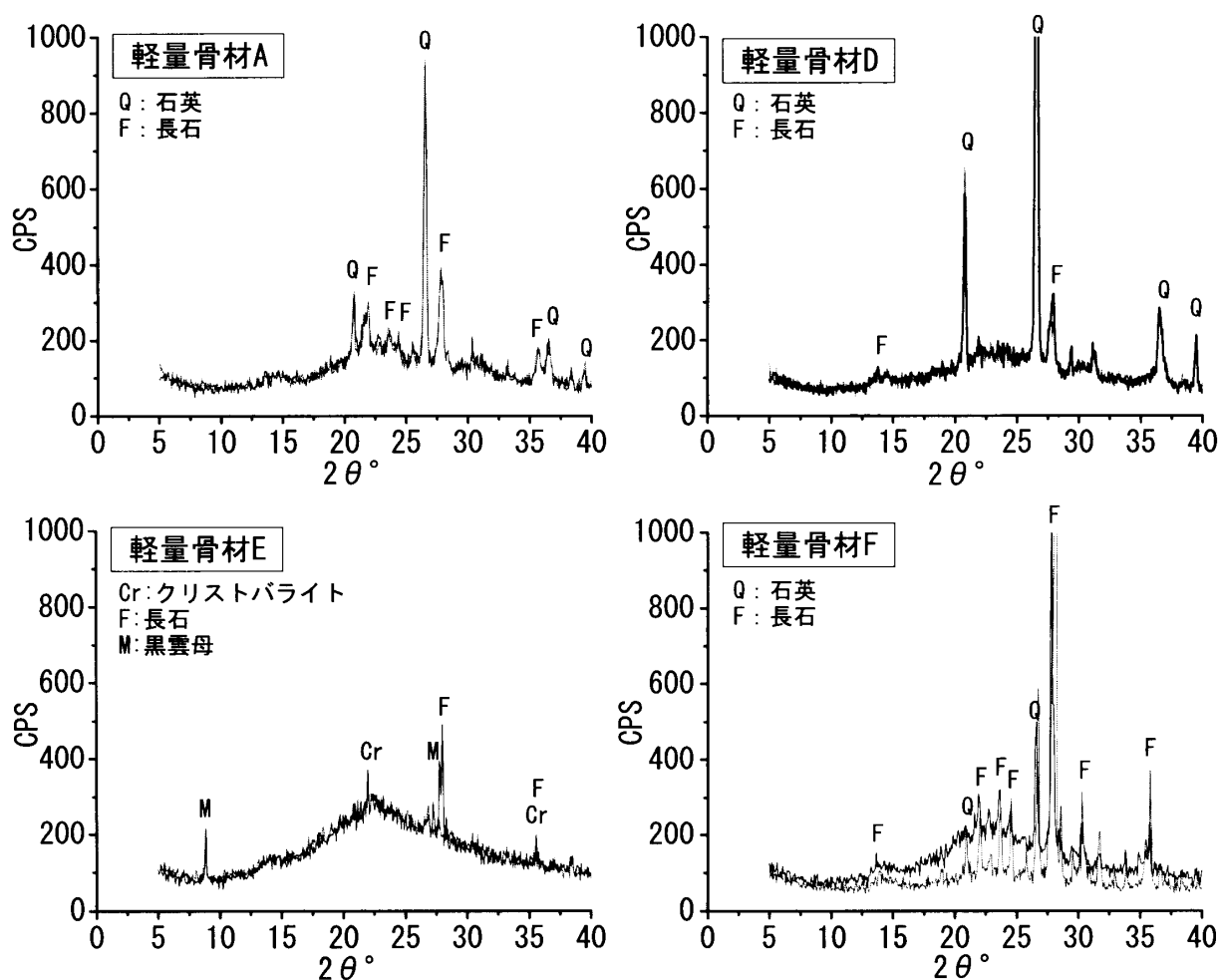
図－1 軽量骨材のX線回折図
