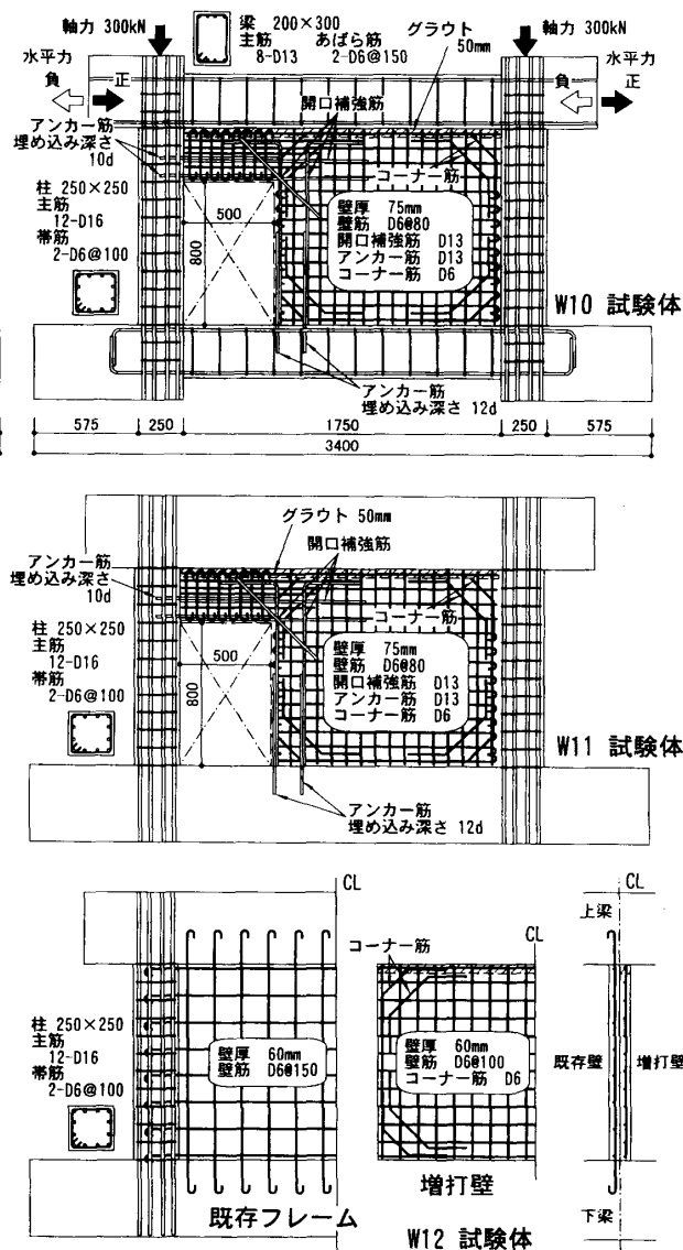
図-2 試験体概要
