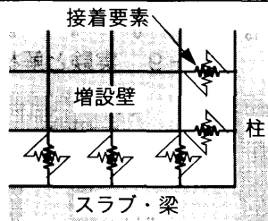
図-7 接着部分のモデル化
