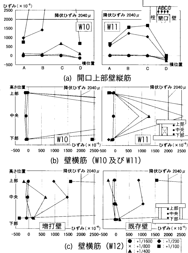
図-5 壁筋ひずみ分布
