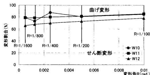
図-4 曲げせん断変形分離
