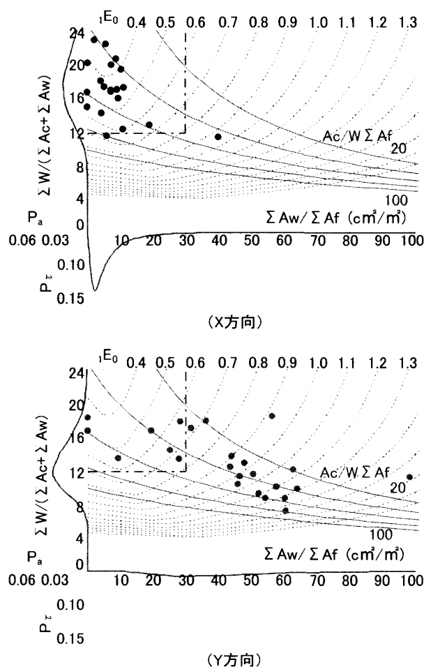
図-4 延床面積壁率と平均せん断応力度の関係
