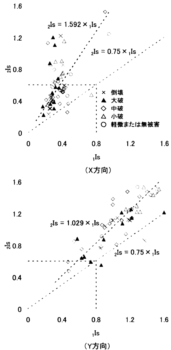
図-6 _1Is と _2Is の関係と地震被害
