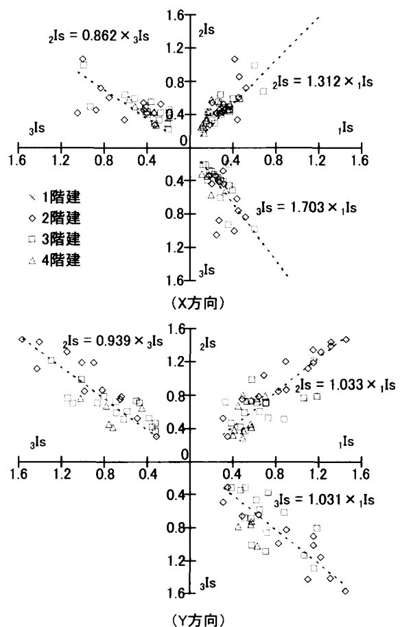
図-3 {}_1I_s - {}_2I_s - {}_3I_s の関係
