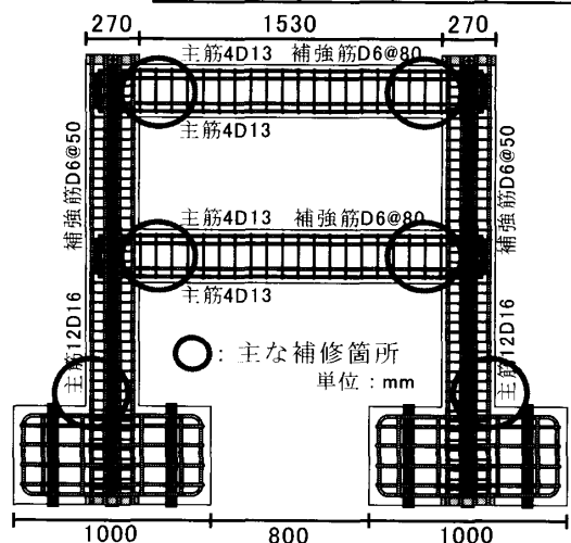
図-1 立面図
