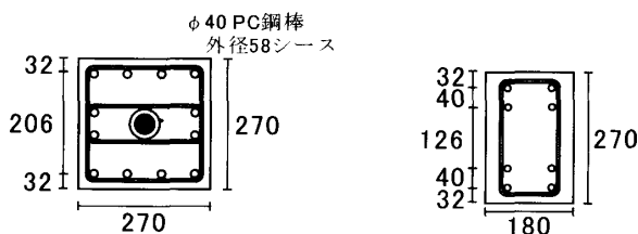
図-2 柱断面図
