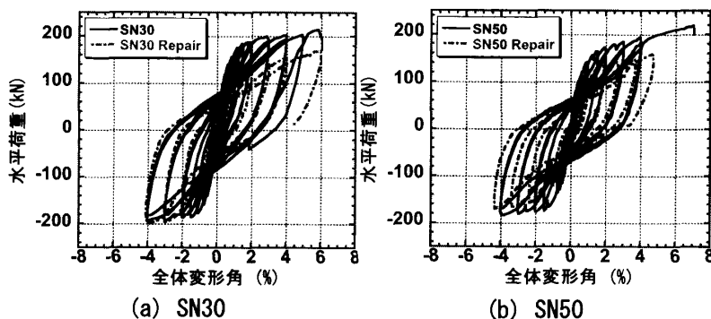
図-8 水平荷重-全体変形角関係
