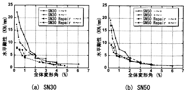
図-9 水平剛性-全体変形角関係
