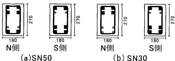
図-4 アンカー差し替え位置（3階梁端）
